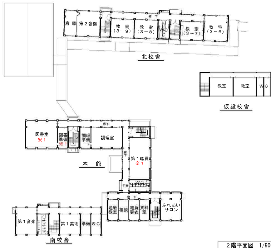
2階平面図 1/900
