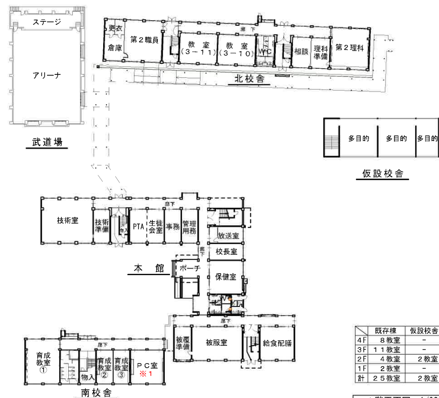
1階平面図 1/900
