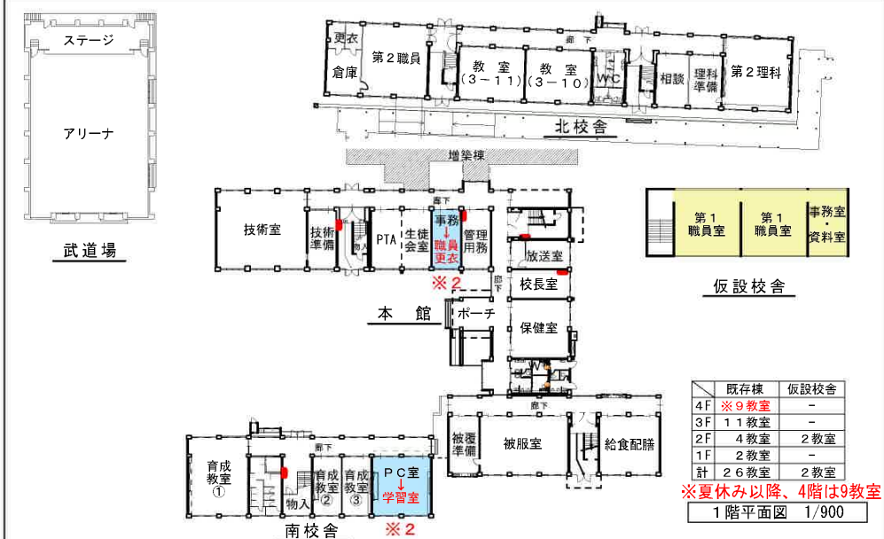
2階平面図 1/900
