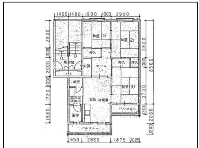
<住戸平面図>
