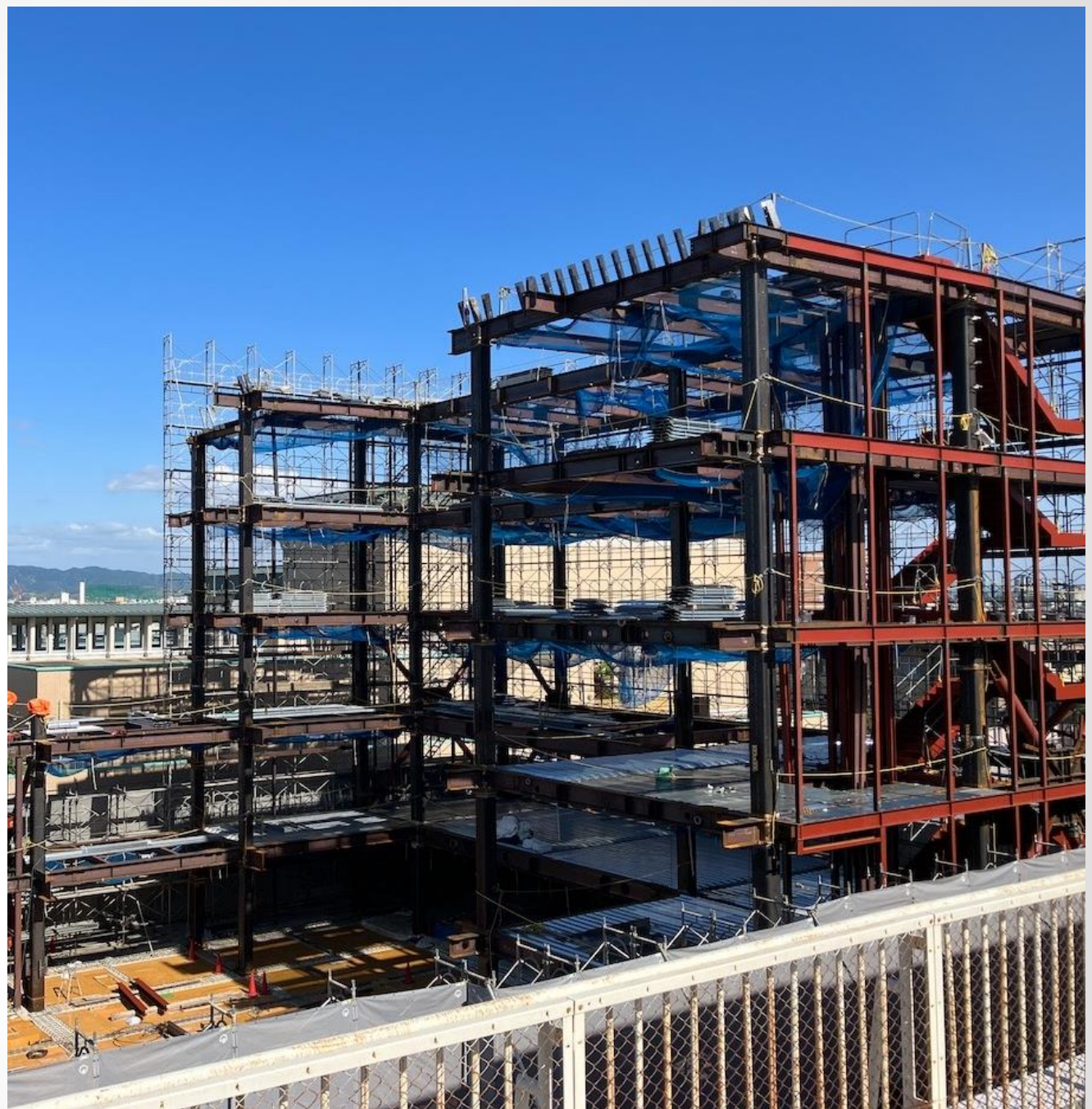
▲鉄骨工事(建て方状況)
