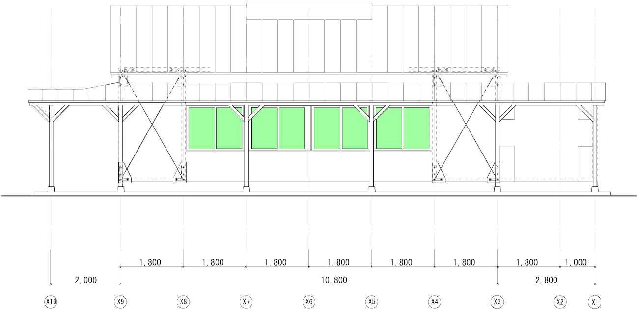
北立面図 1/100
