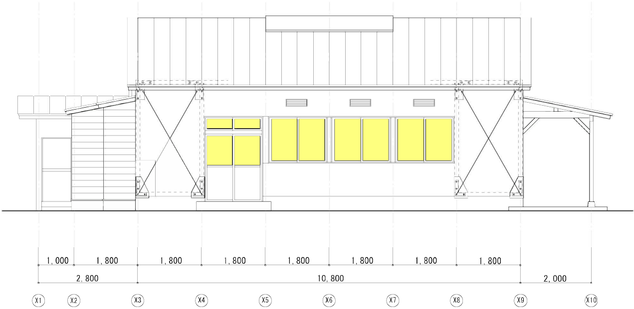
南立面図 1/100
