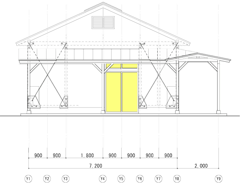
東立面図 1/100
