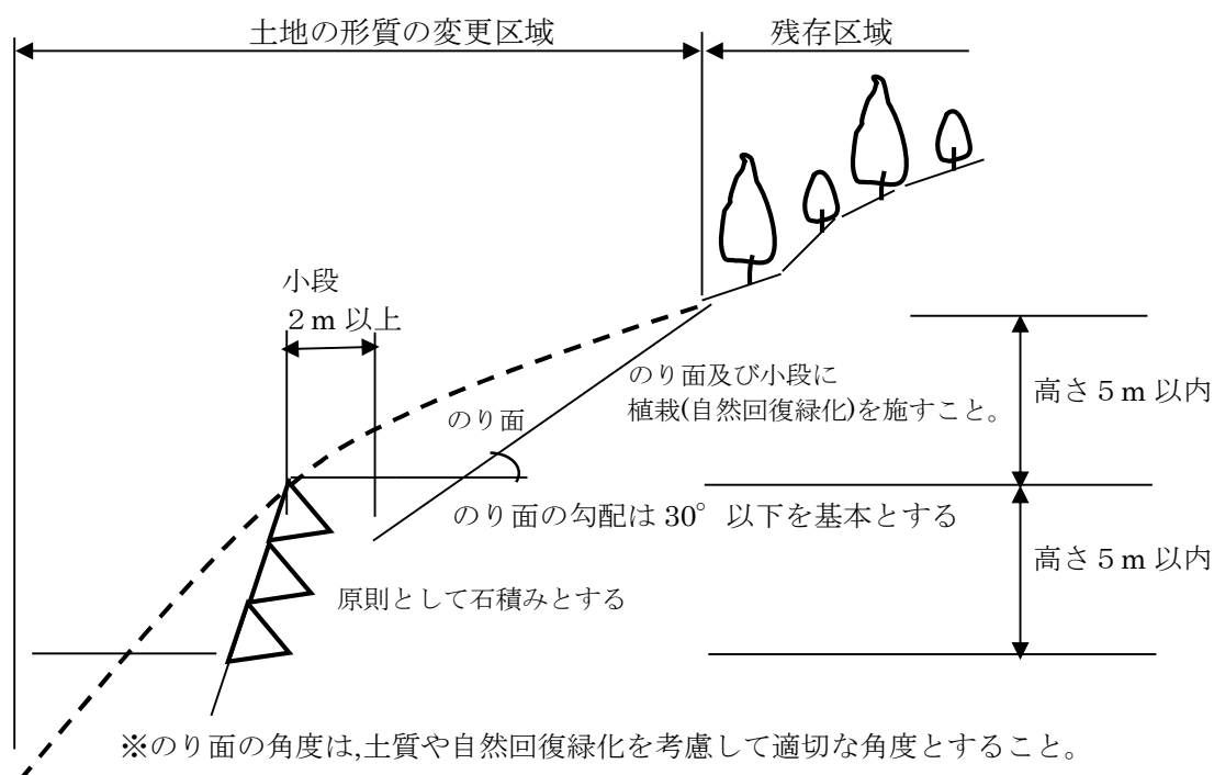
図 1 4 土地の形質の変更におけるのりの例(27ページ関係)
