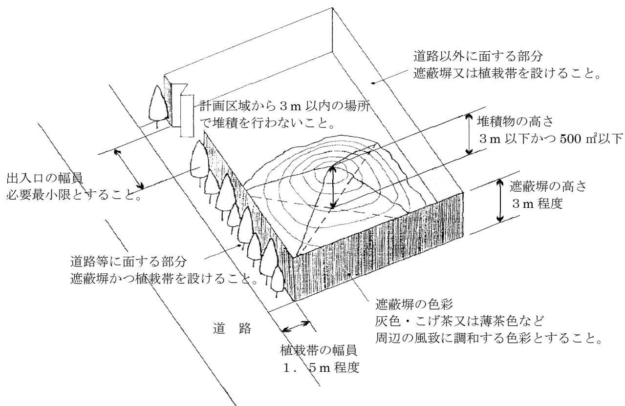
図 1 5 物件の堆積の例と遮蔽のための塀等の例(43ページ関係)
