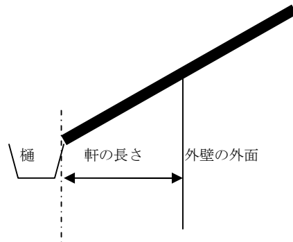
図7 突き出しバルコニーの修景措置の例(20ページ関係)
