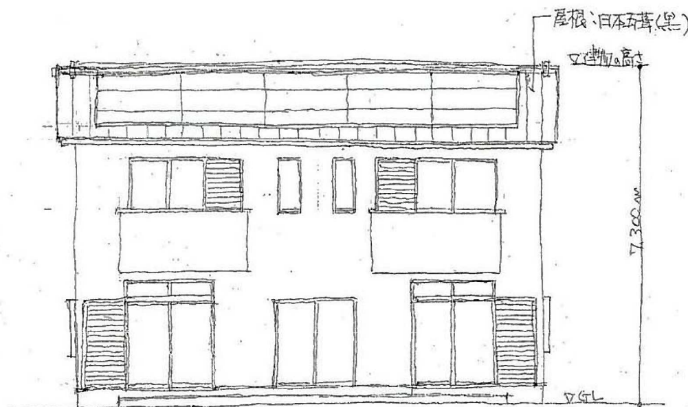
南立面図
