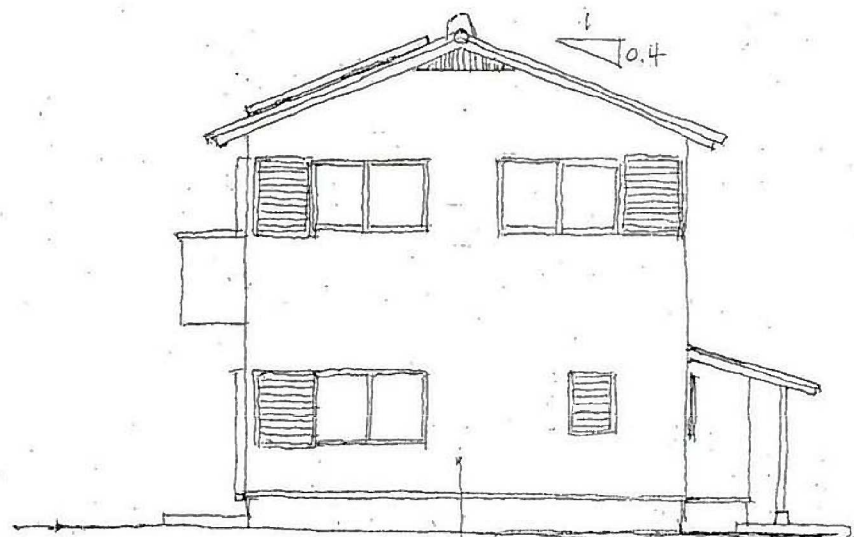
東立面図
