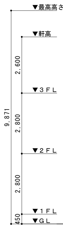
立面図
