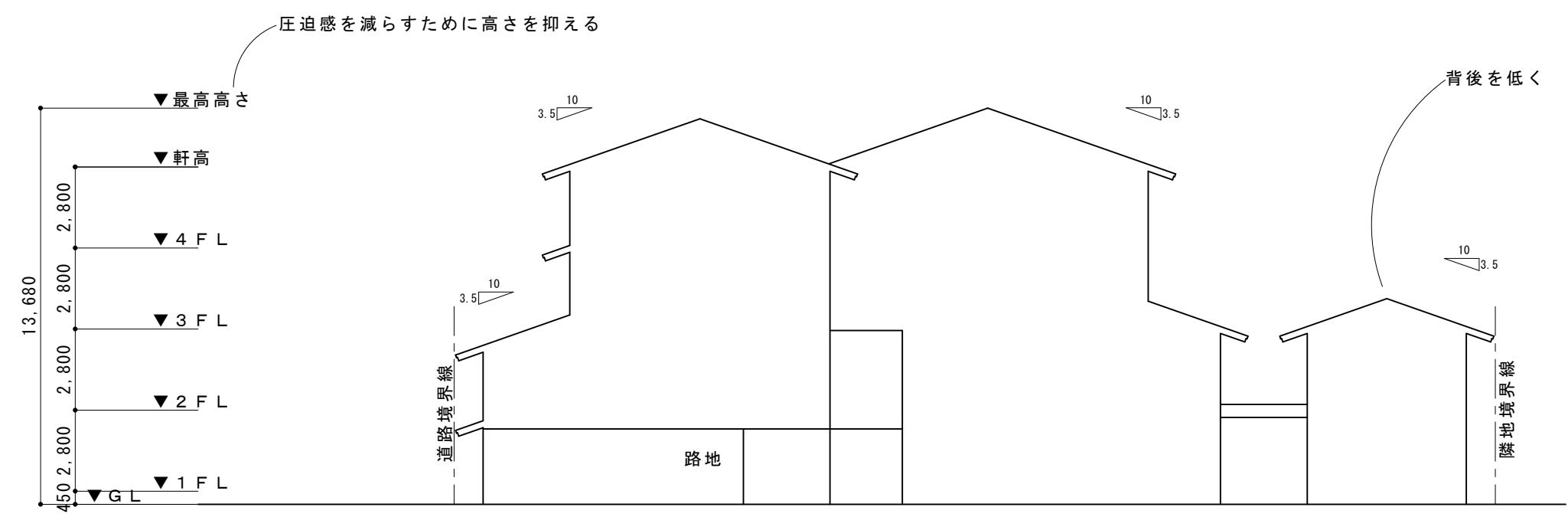
東立面図
