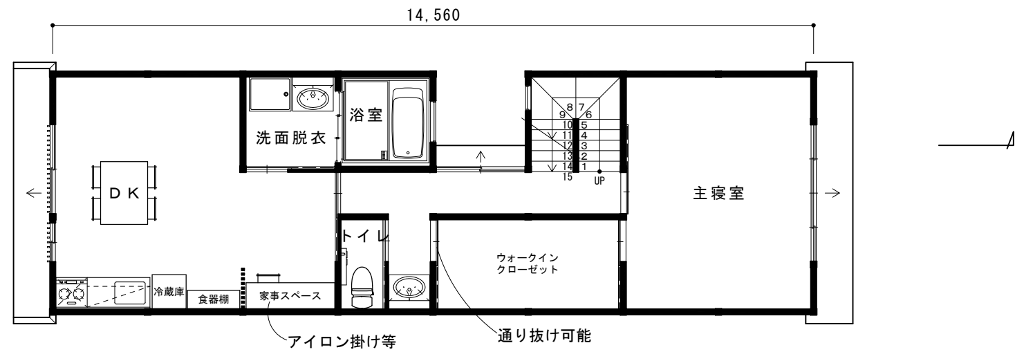
2階平面図
