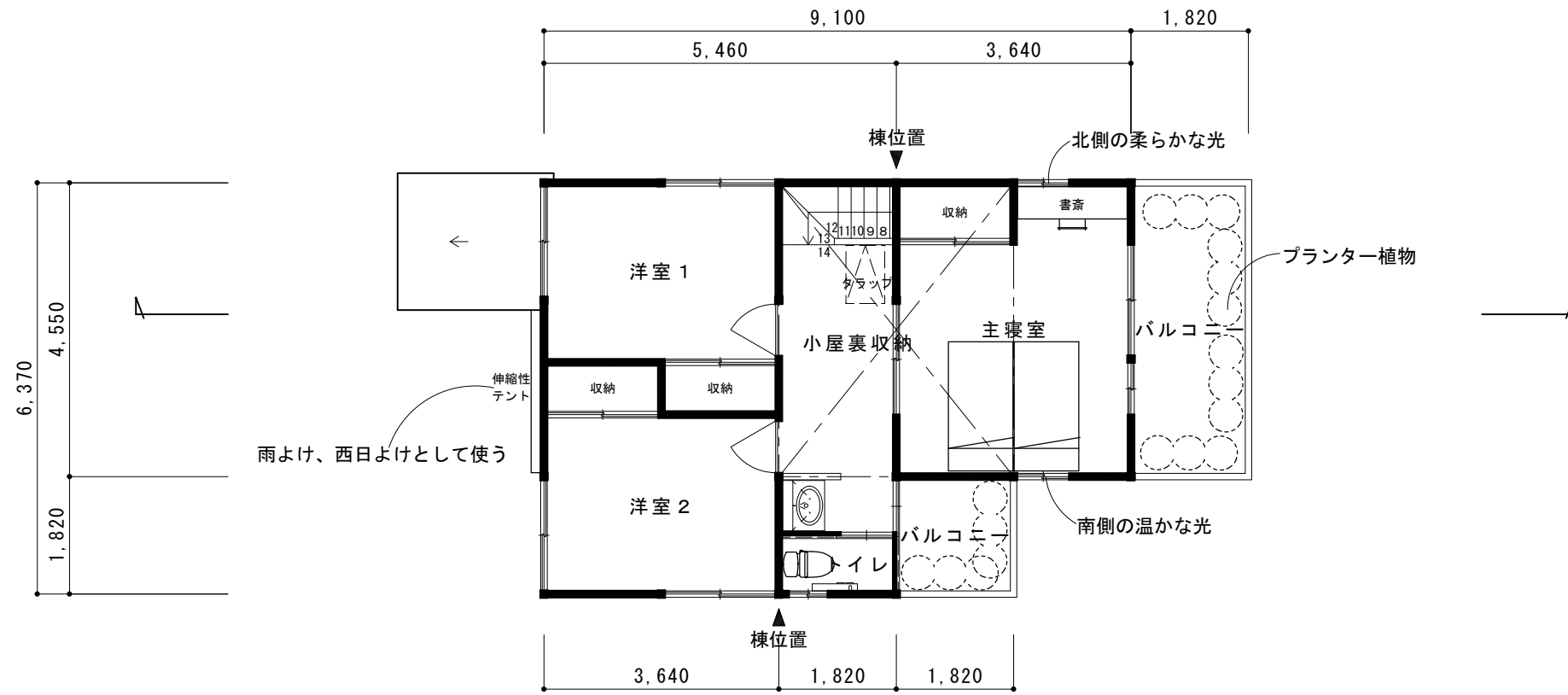
2階平面図
