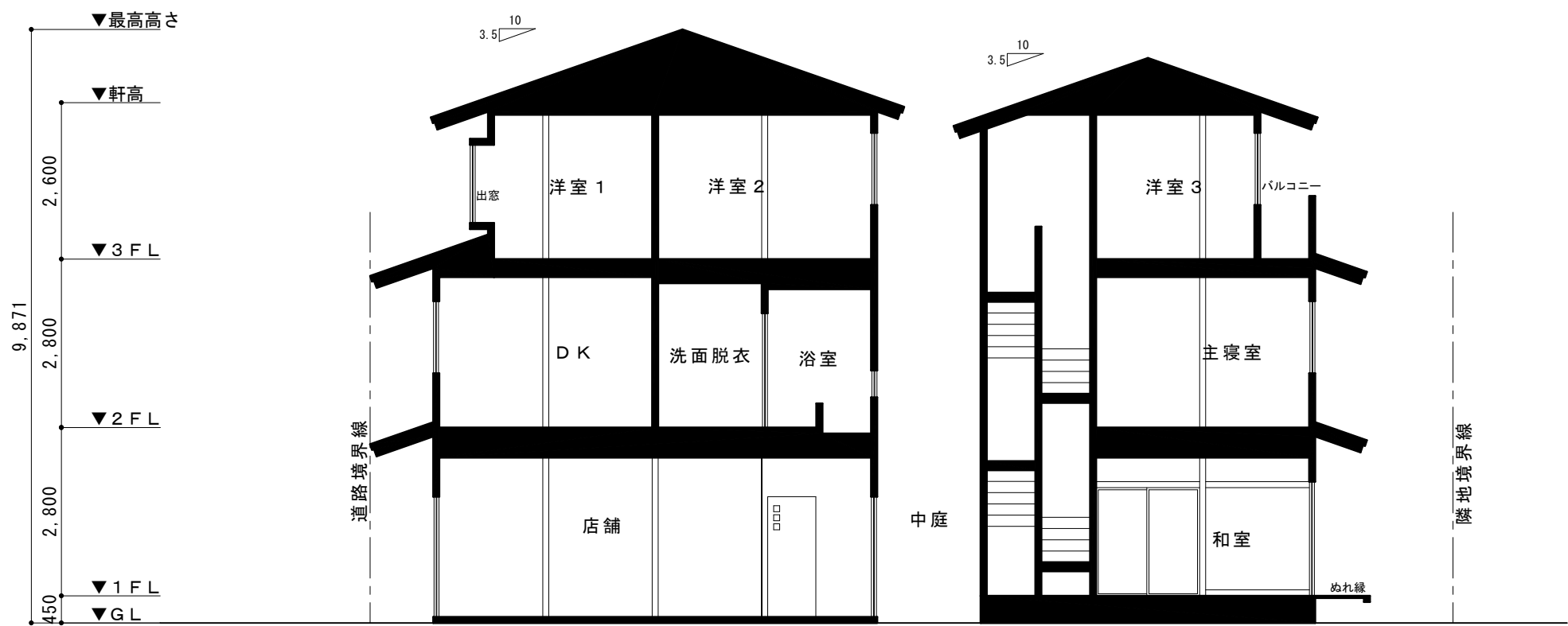
断面図
