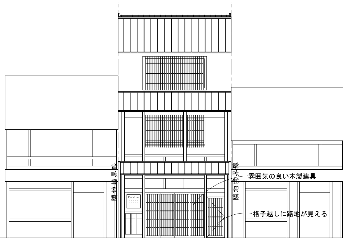
立面図
