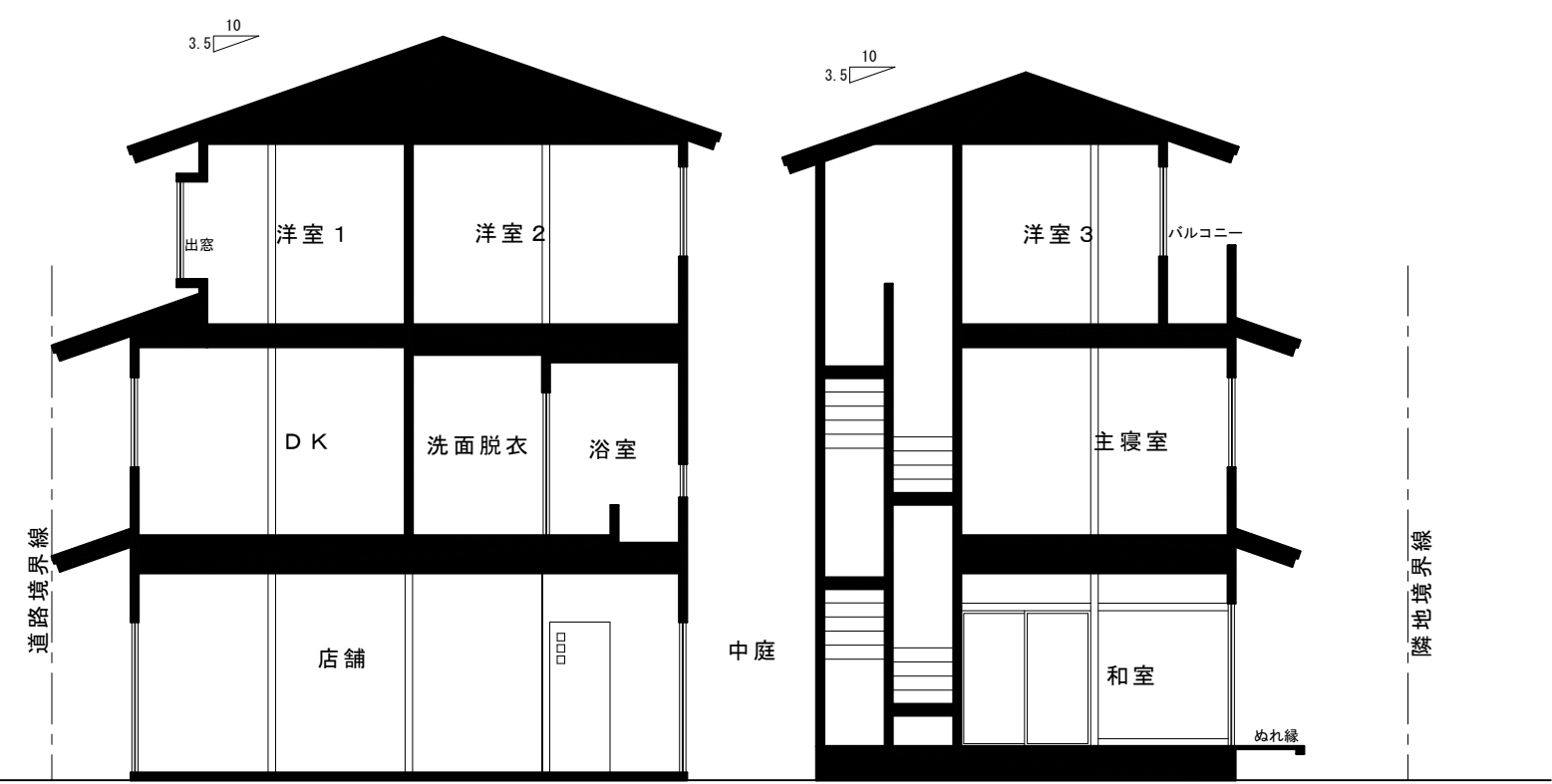
断面図
