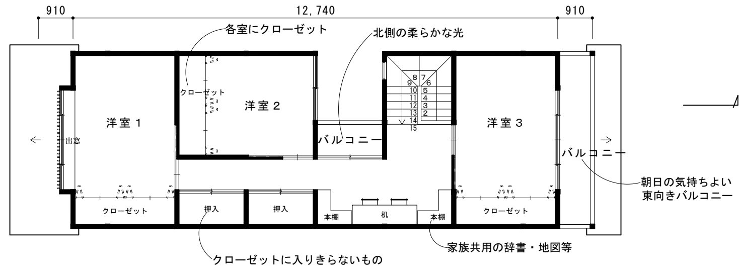
3階平面図
