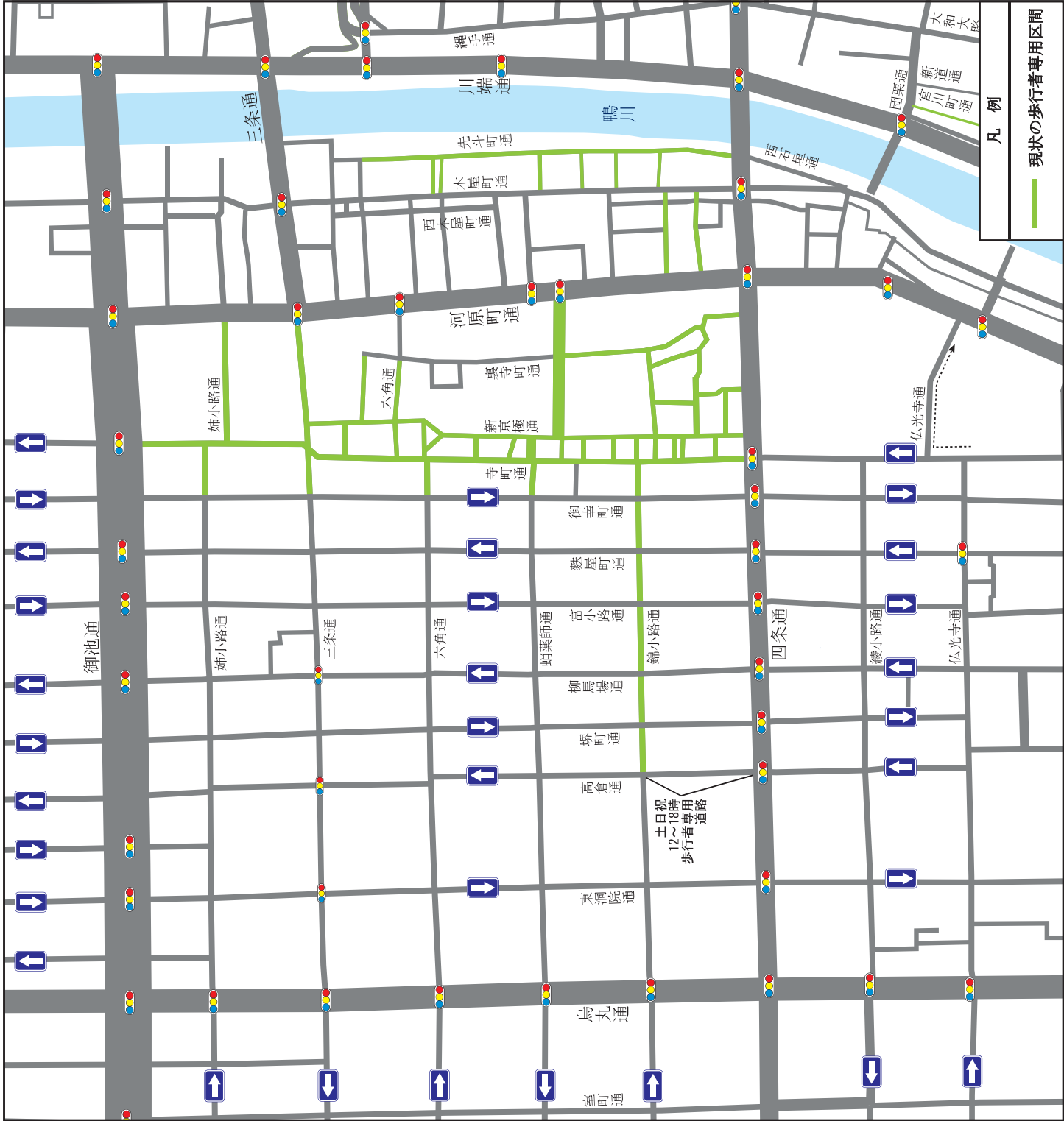
「歩いて楽しいまいまなか戦略」 歴史的都心地区現況図
