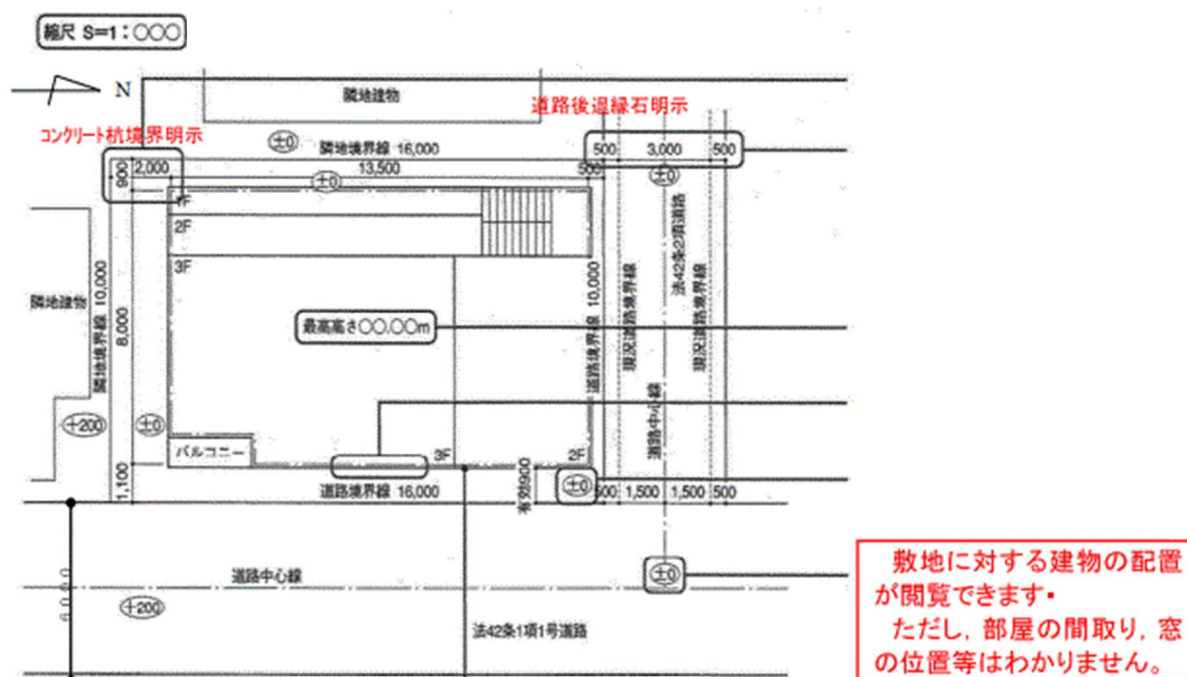
配置図
