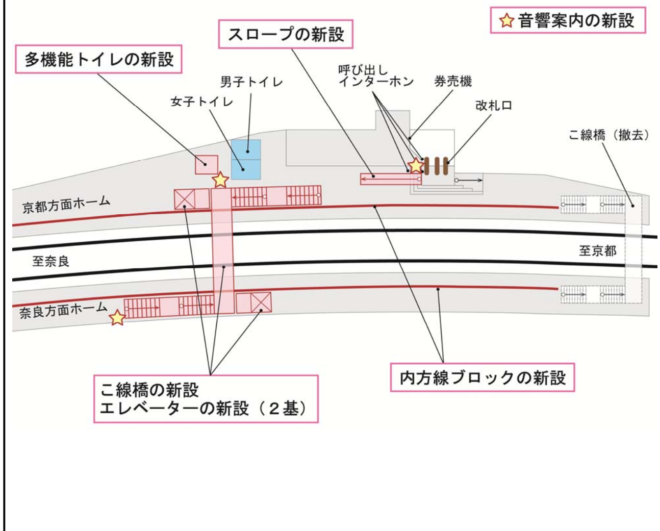
図ー１１ 桃山駅のバリアフリー化の概要
