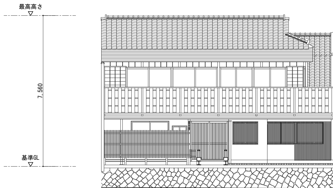
北 立面図
