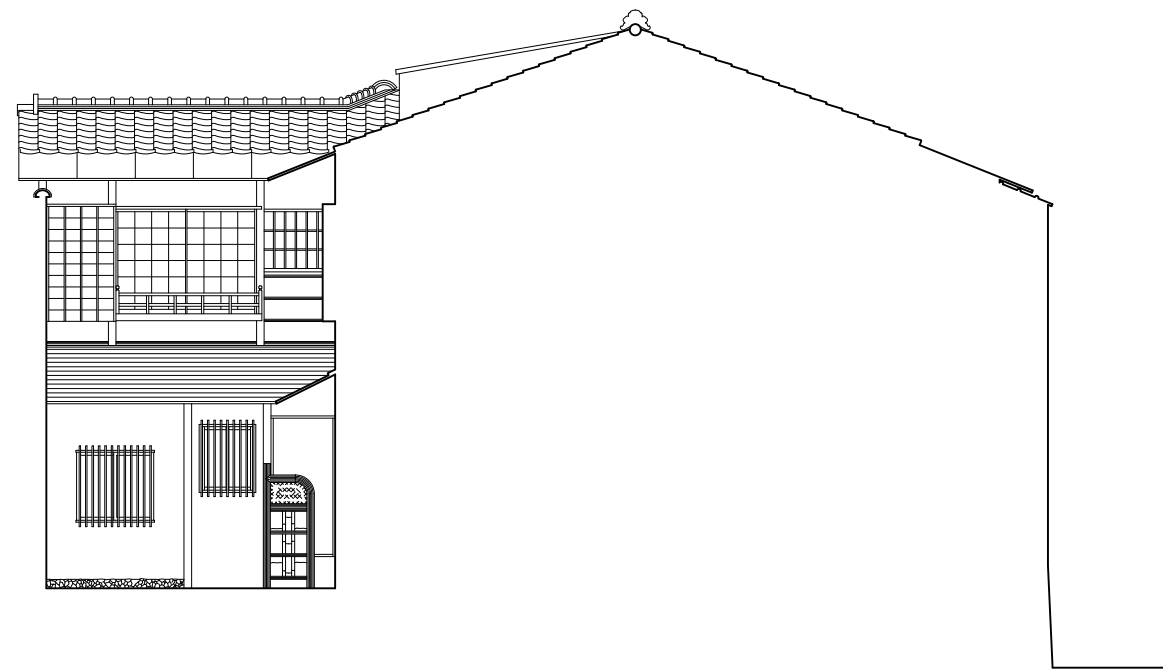
東 立面図
