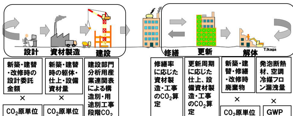
図 4.11 建物の LCA 指針における CO 2 排出量の積上げ(「建設」「修繕・更新・解体」時)
