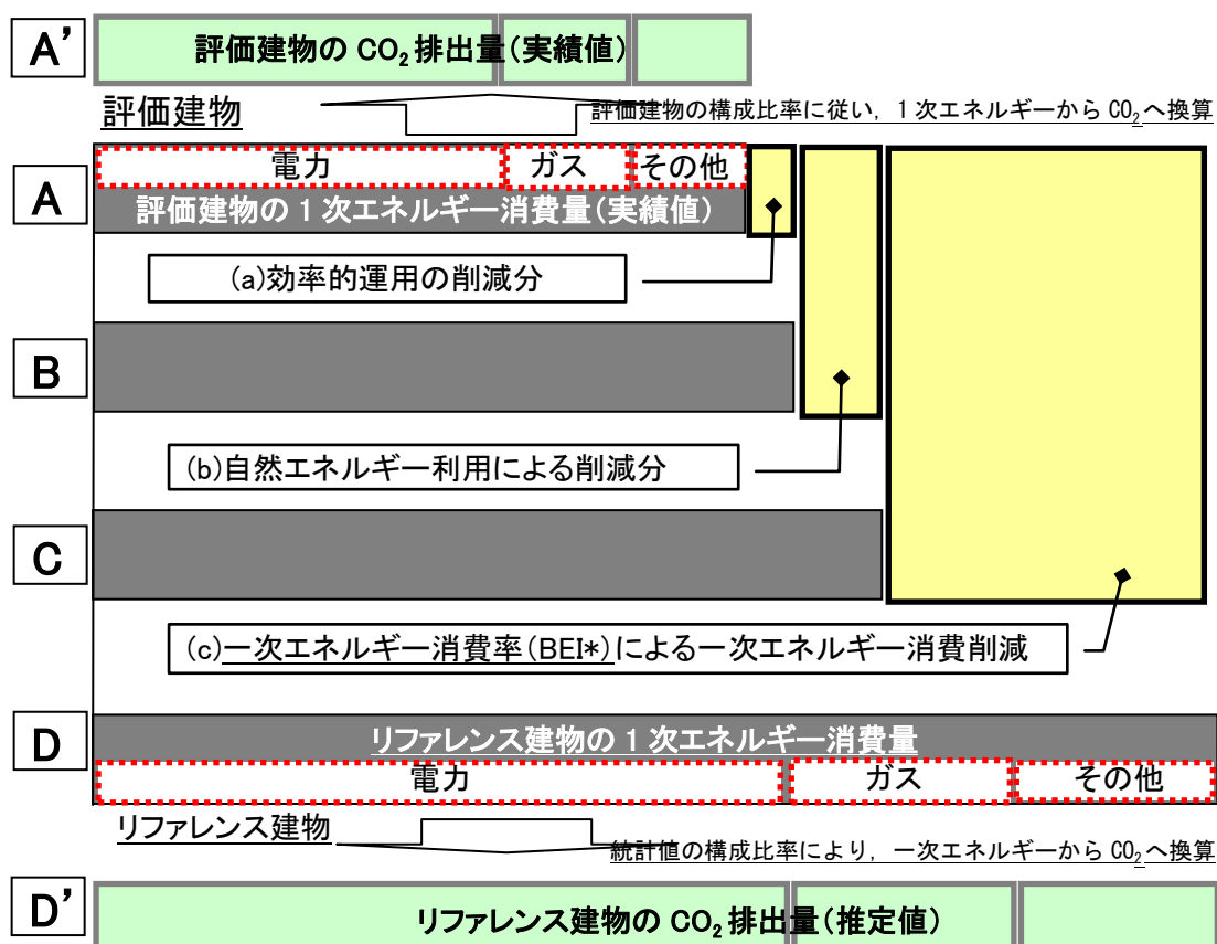
図 4.12 リファレンス建物の CO 2 排出量算定の考え方
