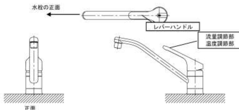
図 水優先吐水機構—台所水栓(正面で湯が吐出しない構造)の例
