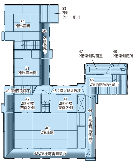
主屋2階平面図
