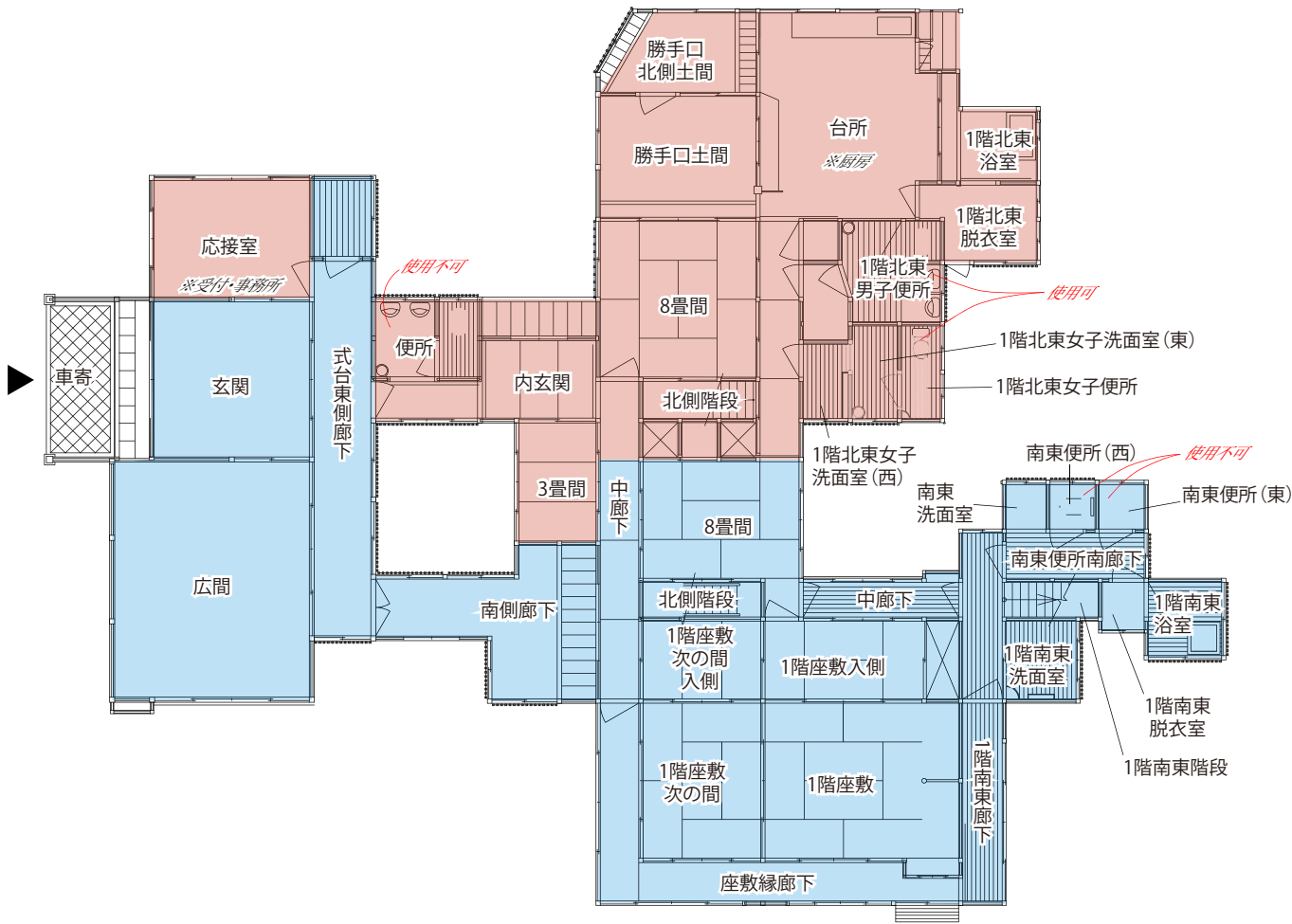
主屋1階平面図
