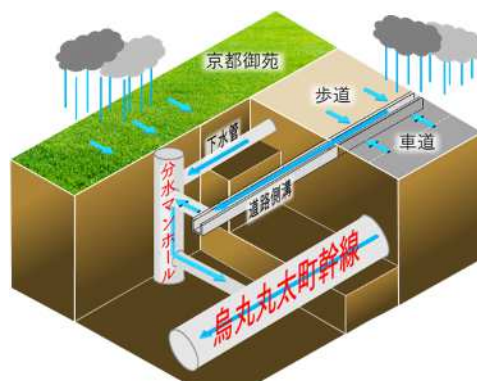
幹線内への雨水取込みイメージ
