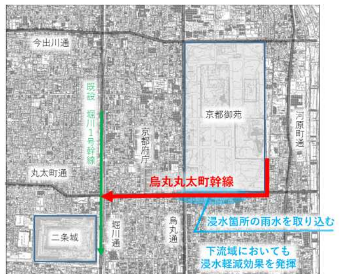
幹線整備位置図
