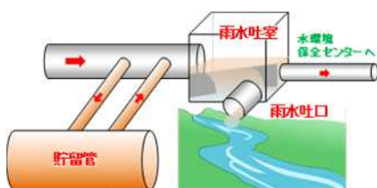
貯留管による対策イメージ
