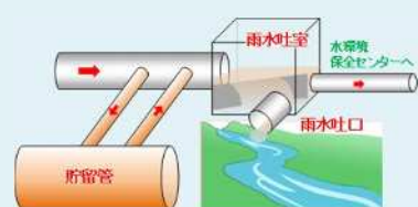
一時的に貯留する施設を整備 貯留管による対策イメージ
