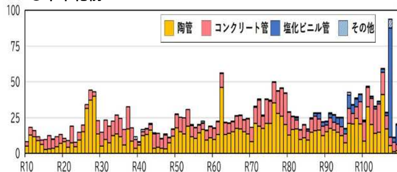
【下水道管路の更新需要（100年間）】
