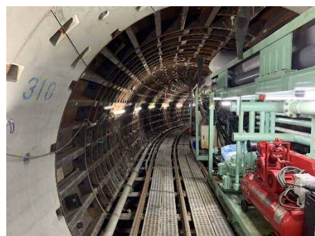
新山科浄水場導水トンネル築造工事 （トンネル掘進の様子）
