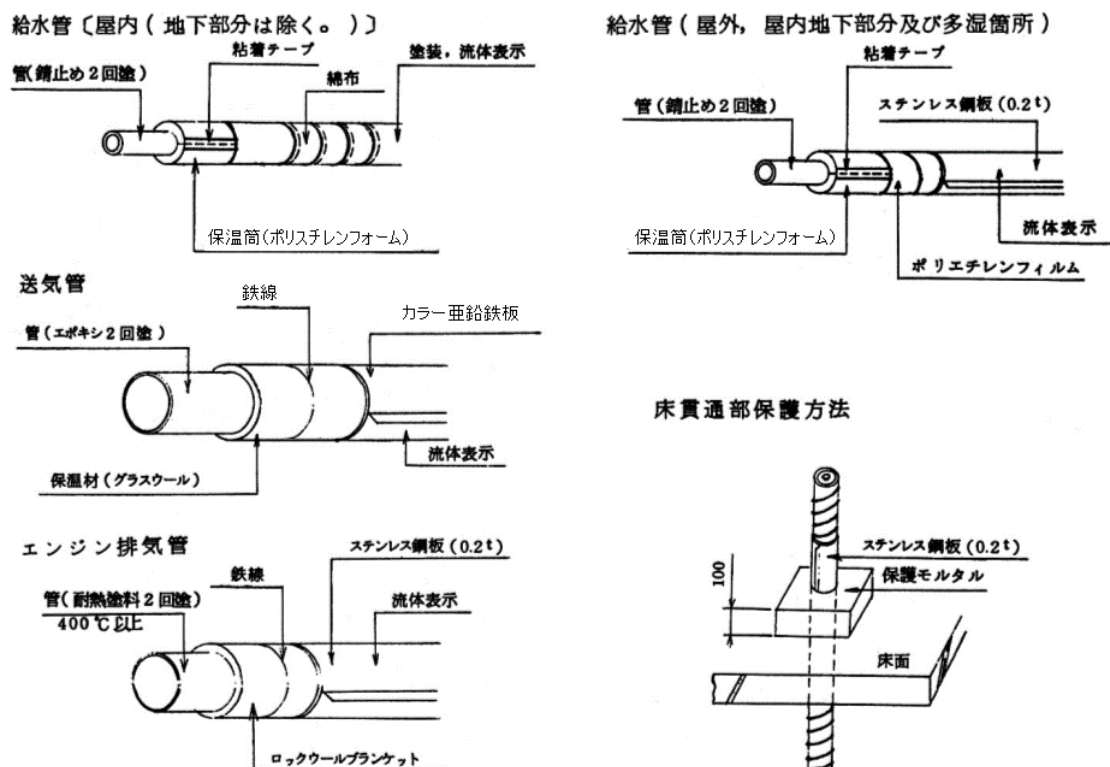
図 3-6 標準図
