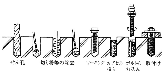
図1-4 接着系アンカーの施工の例
