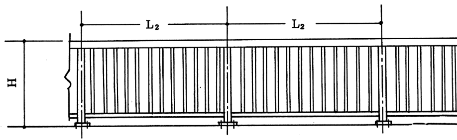
図 1-2 アルミ製手すり
