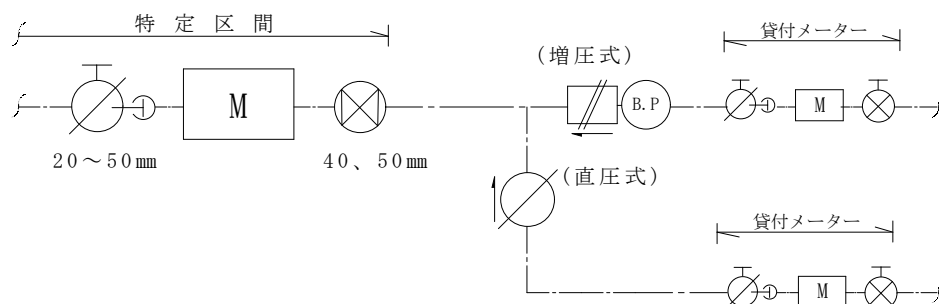
直結ゾーニング式50mm以下
