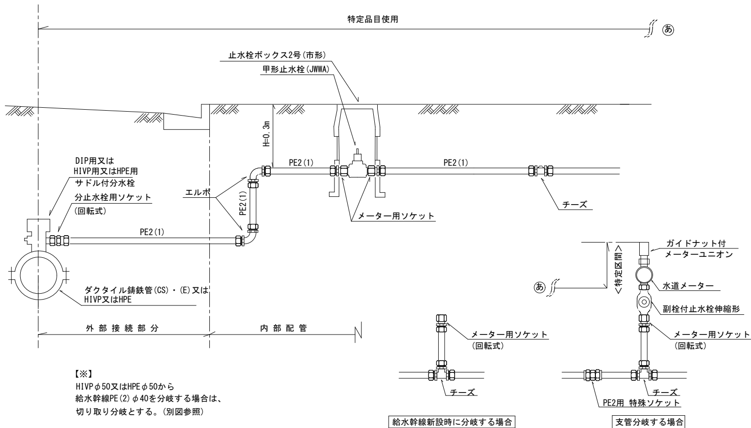
図名 給水幹線標準配管図(旧京北地域水道) 京都市上下水道局水道部水道管路課
