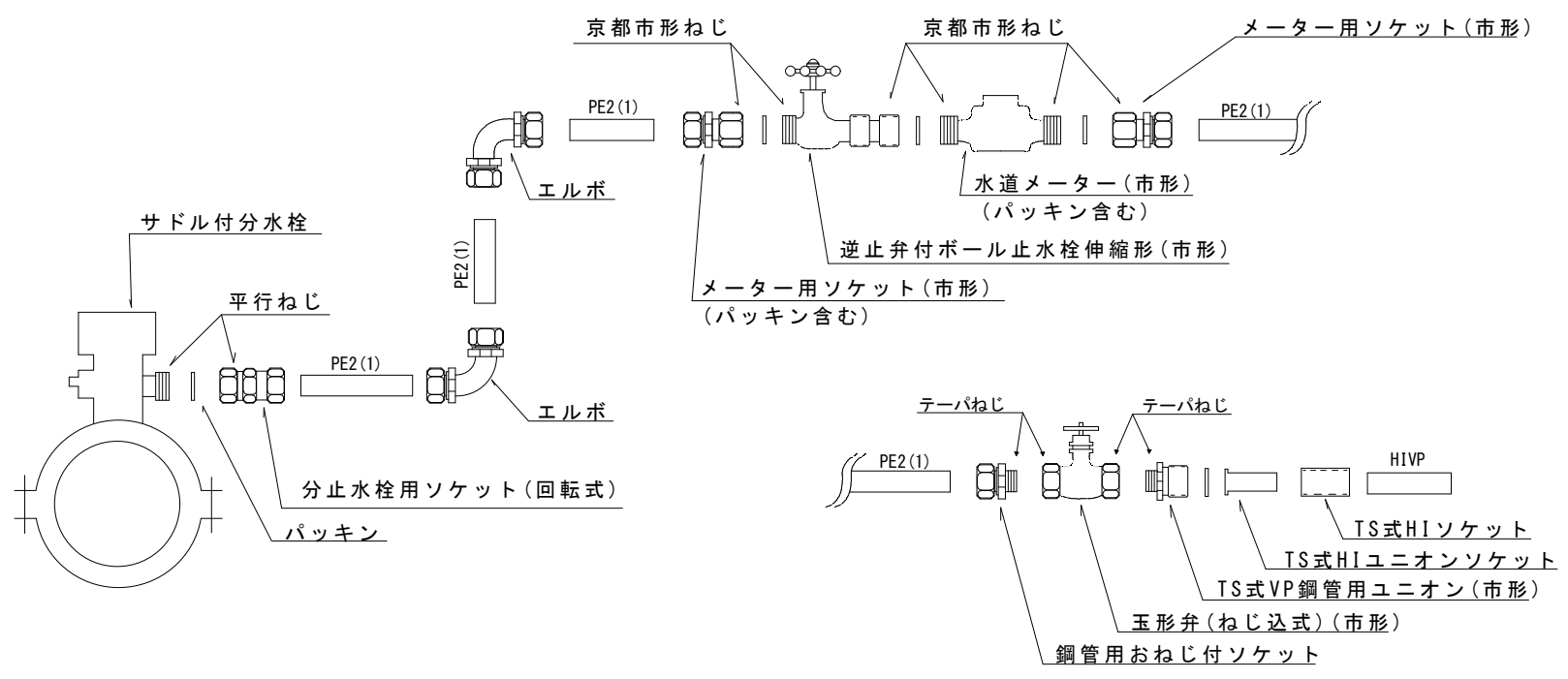
図名 給水装置標準配管概略図 適用 一般個人住宅及び受水槽式 φ 40 mm 京都市上下水道局水道部水道管路課
