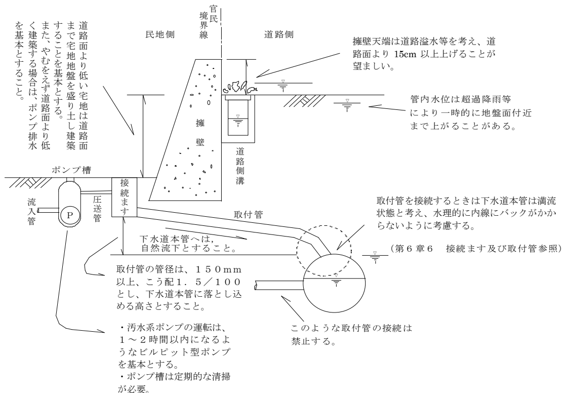
図 3-2 1 道路面より低い新築家屋計画時の注意点
