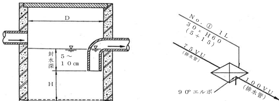
図 3-11 1 L 型トラップます (鉄筋コンクリート製)
