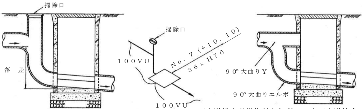
(2) ドロップますの例 (プラスチック製)
