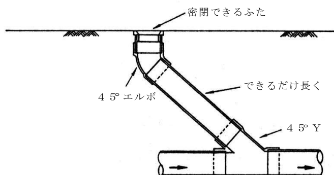
図 3—1 3 掃除口の例（ますが設置できない場合）
