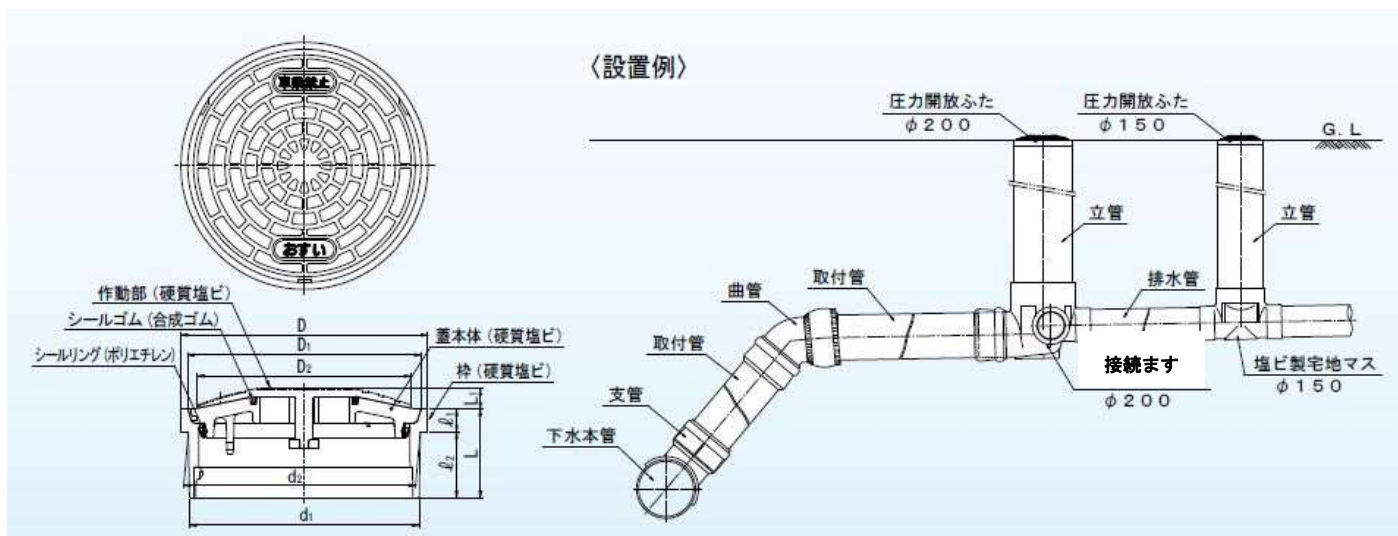
図 3－2 2 逆流防止等措置の例（圧力開放ふたの設置）
