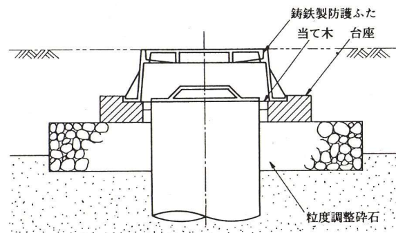
図 3-4 防護ふたの例
