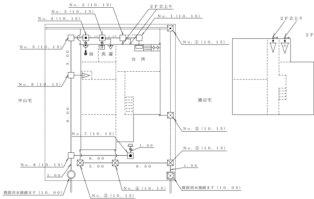
図 3－17 平面図（配置図）の例
