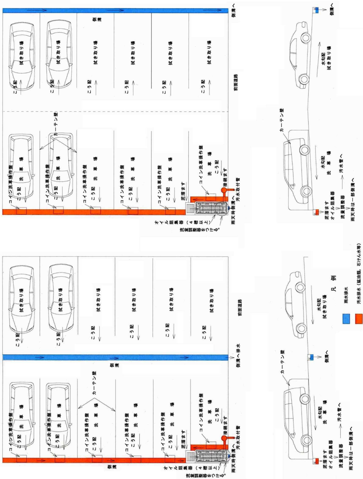
図3—28 洗車場排水の例
