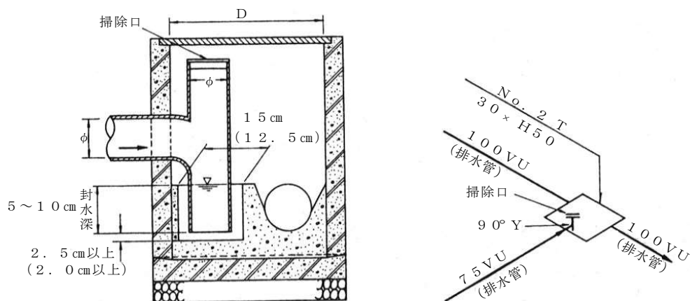
図 3－9 T型トラップますの例（鉄筋コンクリート製）
