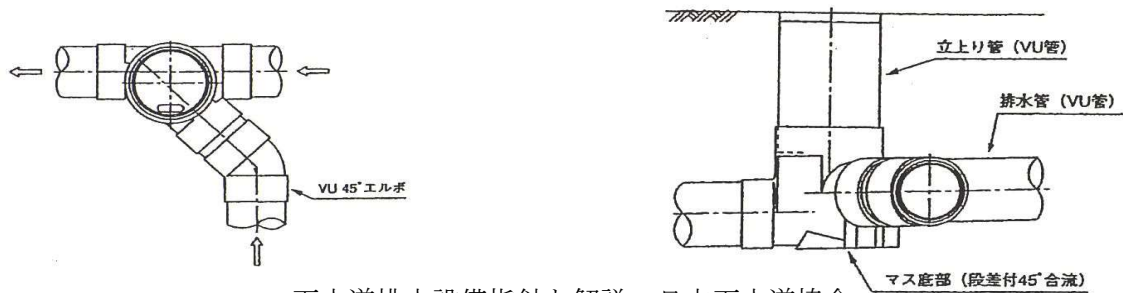
図 3—6 便所からの排水が直接流入するますの例
