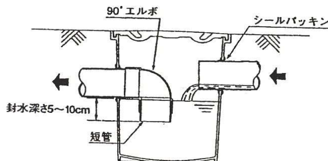
図 3-12 1 L型トラップます (ポリプロピレン製)
