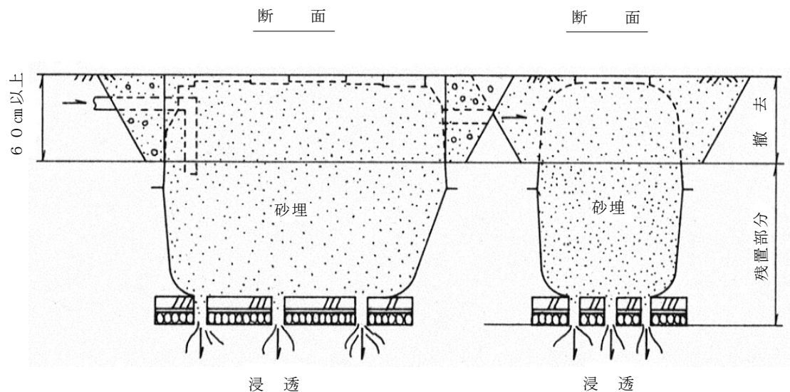
図 3—30 浄化槽撤去例
