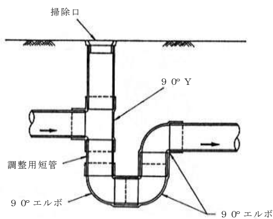
図 3—1 4 トラップ付掃除口の例 (器具トラップ又はトラップますが設置出来ない場合) トラップ式掃除口 (内径式)
