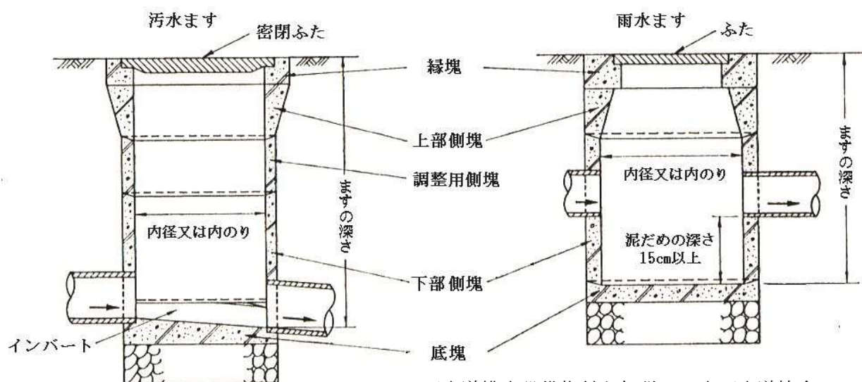
図 3—3 ますの例 (1) 既製ブロックますの使用例
