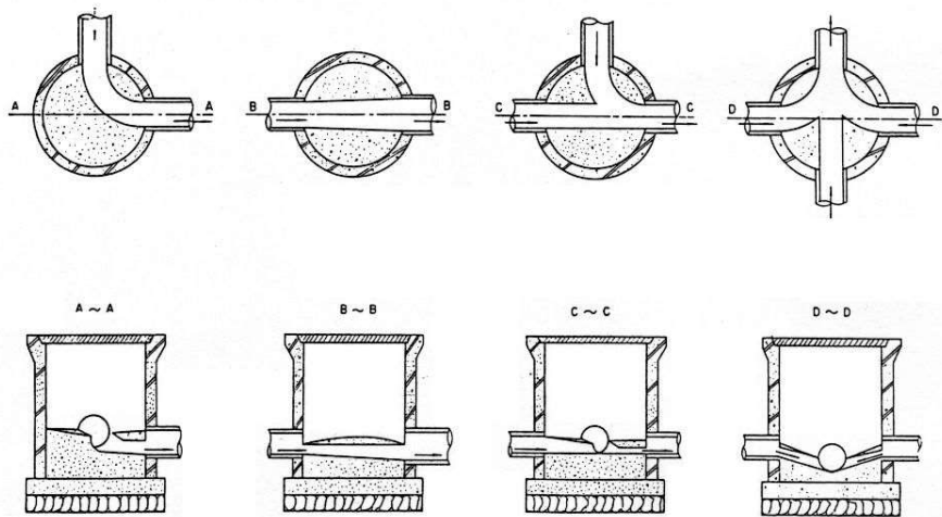
図 3-5 インバートの施工例
