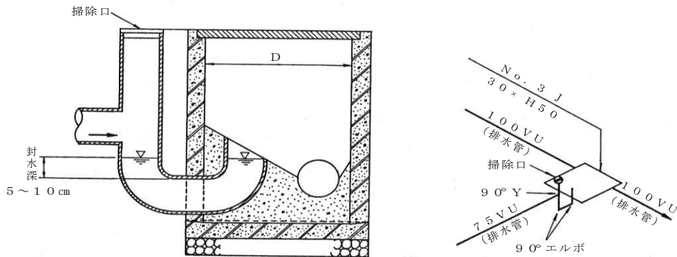
図 3-10 J 形トラップますの例
