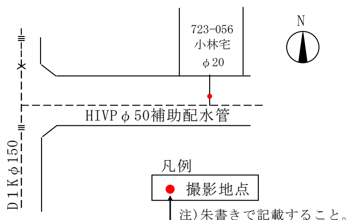
給水装置工事の見取図
