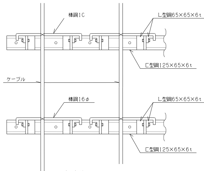
A-A 断面図
