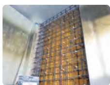
配水池の耐震化工事
