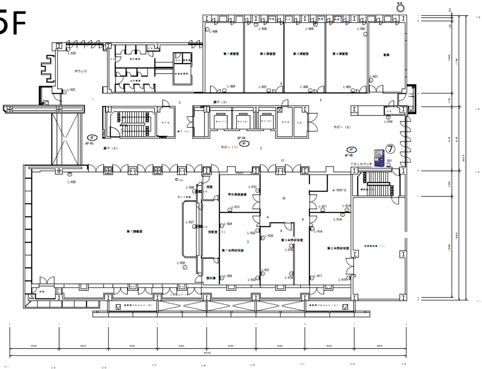
5層 平面図
