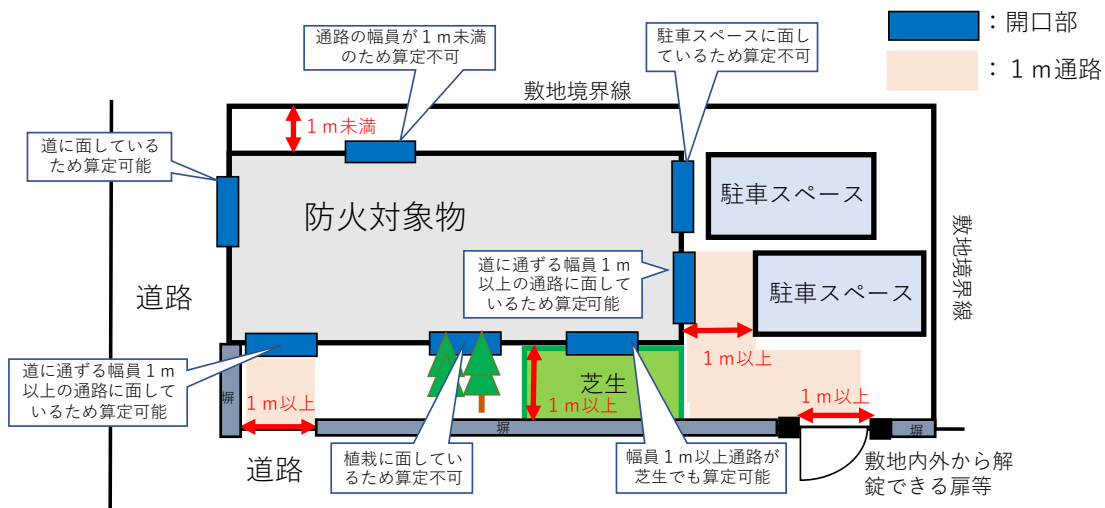
図3 道又は道に通ずる幅員1m以上の通路その他の空地の例
