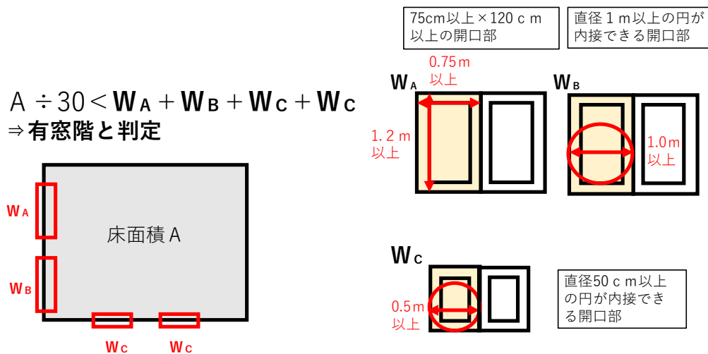
図1 有窓階と判定できる例
