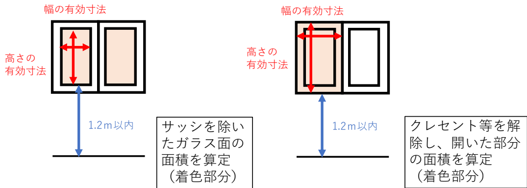
図5 はめごろしの窓等とクレセント付きの窓等
