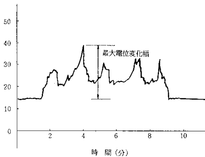
地表面電位測定例
