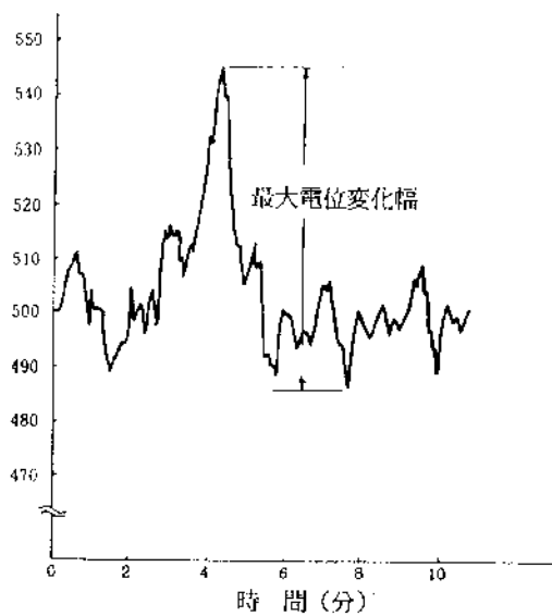
対地電位測定例
