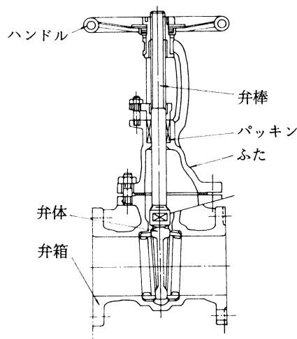
仕切弁の例
