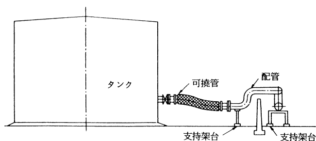
立面図
