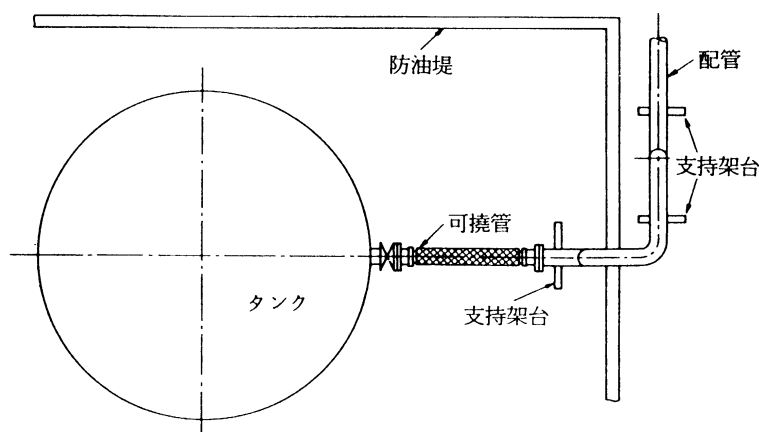
平面図
