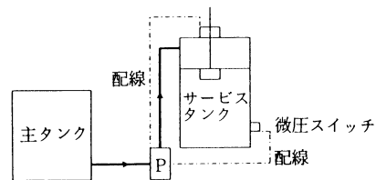
フロートスイッチと微圧スイッチ
