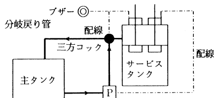
フロートスイッチと分岐戻り管等
