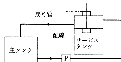
フロートスイッチと戻り管
