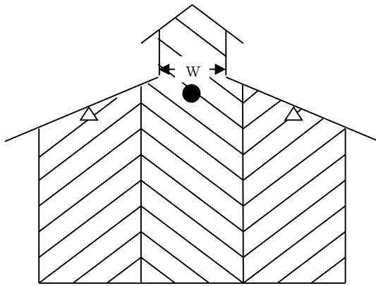
第24-104図 断面図
