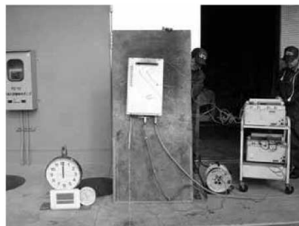
ガス給油器の再現実験
