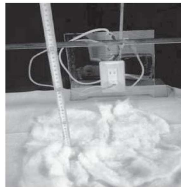
短絡痕による可燃物への着火実験
