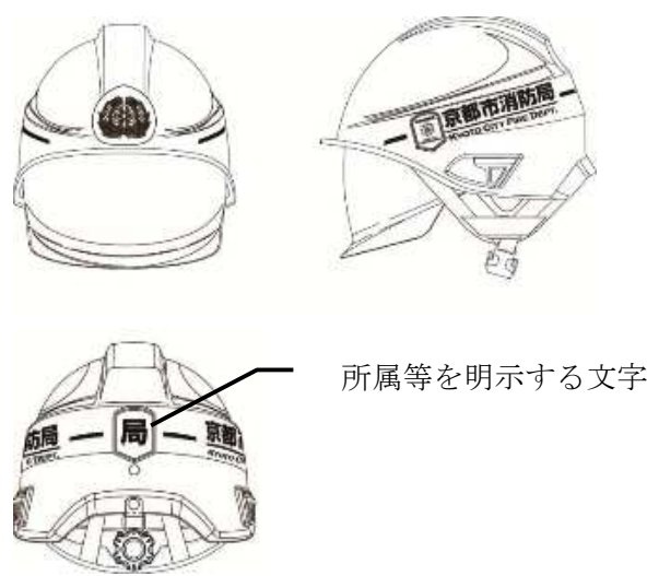
防火帽制式の図
