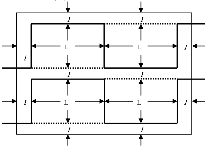
第24-64図 一边省略の例2
