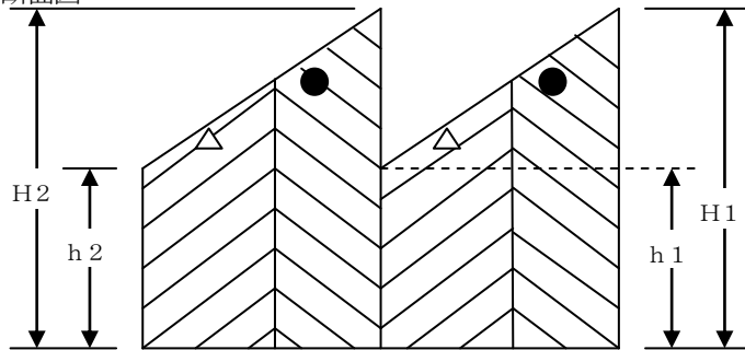
第24-98図 断面図
