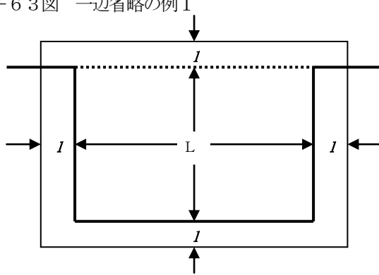
第24-63図 一边省略の例1
