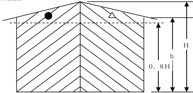
第24-97図 断面図
