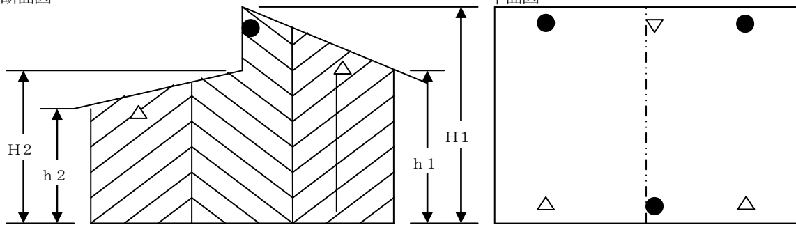
第24-100図 断面図
