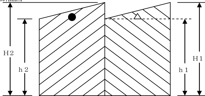
第24-99図 断面図
