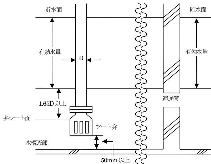
第13-6図 <サクシヨンピットを設けない場合又は連通管を設ける場合>
