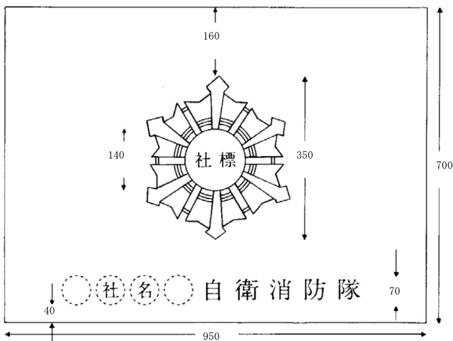
図 自衛消防隊旗 形状 (単位 ミリメートル)
