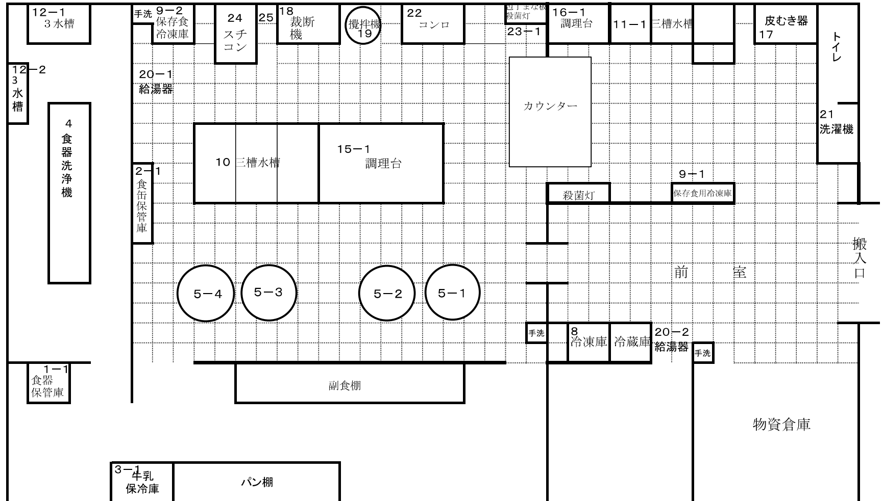
京都市立大枝小学校 給食室配置図
