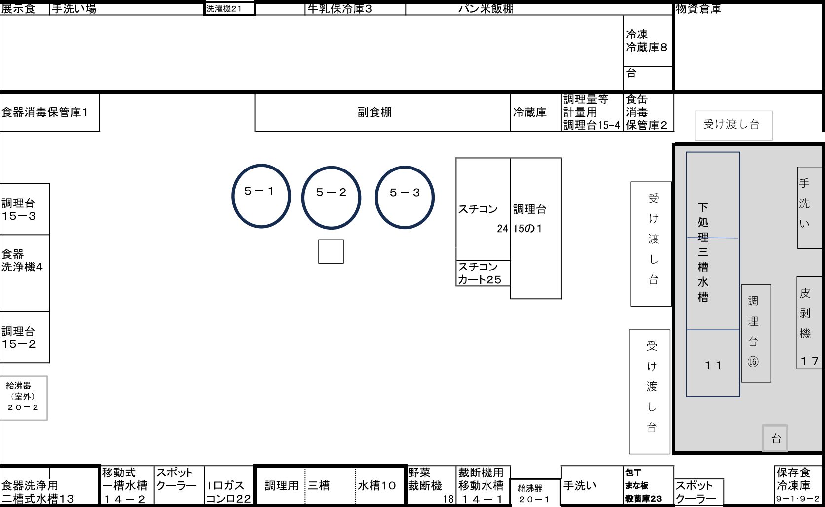
大原小中学校 給食室平面図
