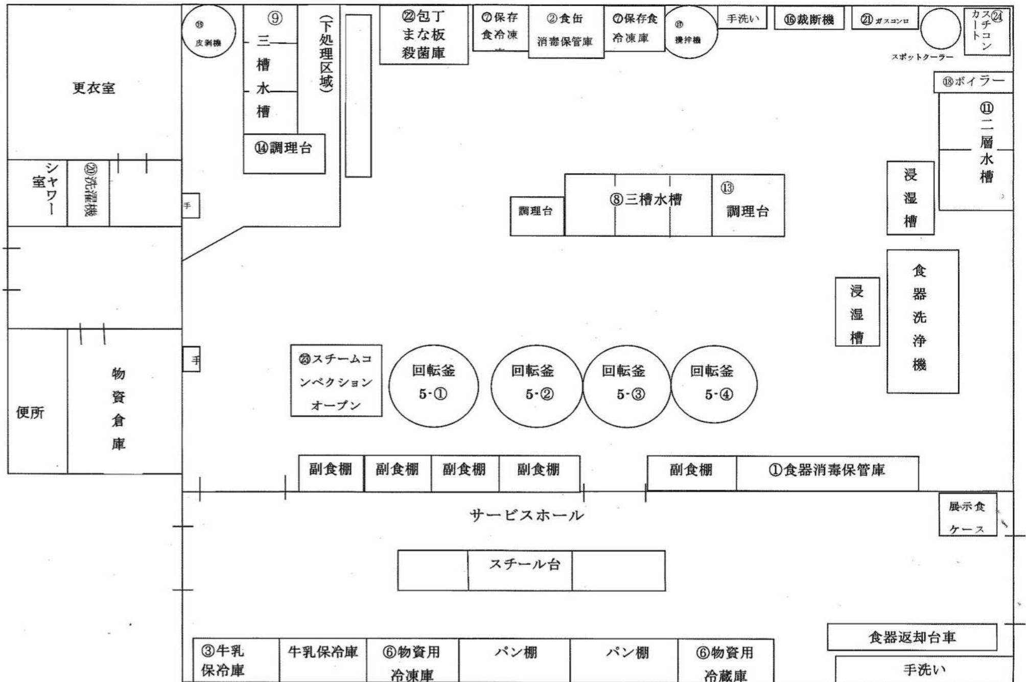
京都市立美豆小学校給食室平面図
