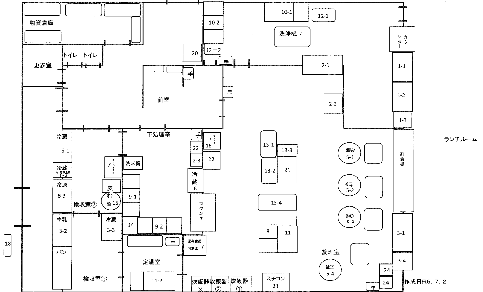
京都市立京都京北小中学校 平面図
