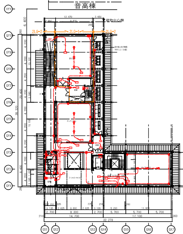
2階平面図
