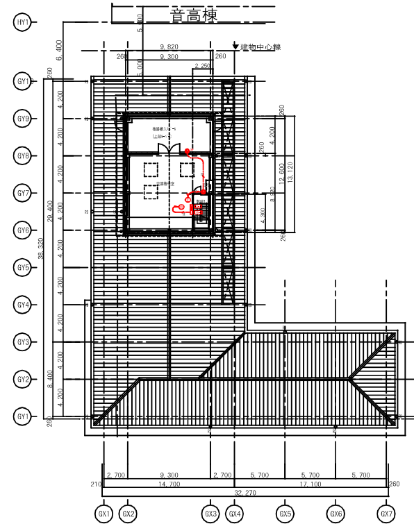
PH階平面図
