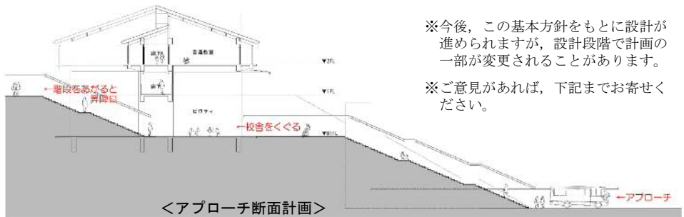
＜アプローチ断面計画＞
