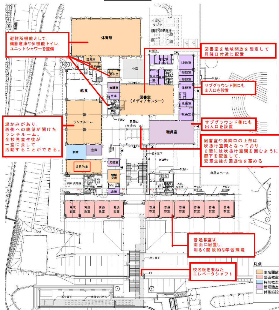
1階平面図
