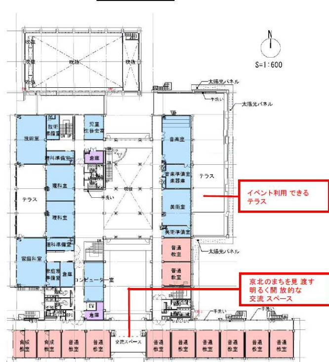
2階平面図
