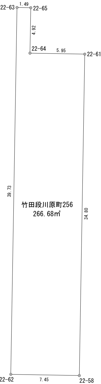
座 標 求 積 表
