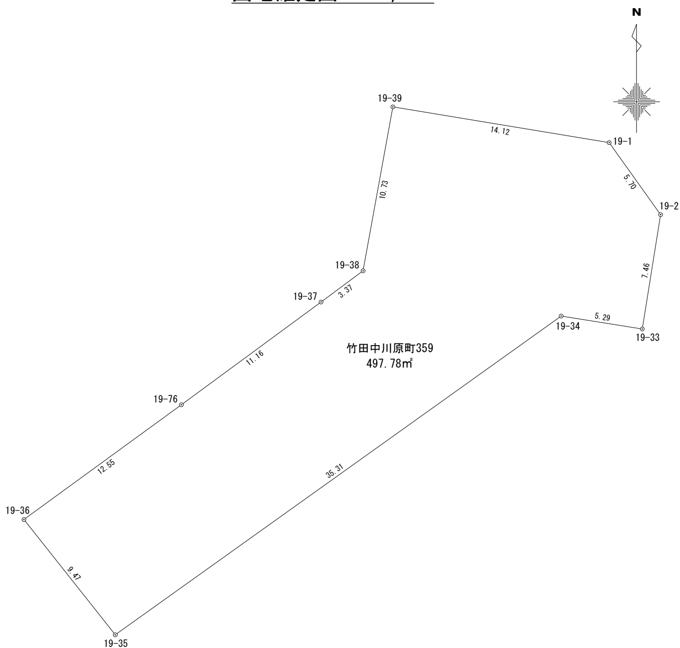
座 標 求 積 表
