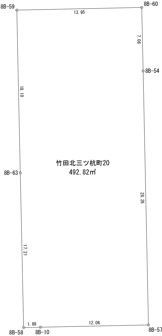
座 標 求 積 表
