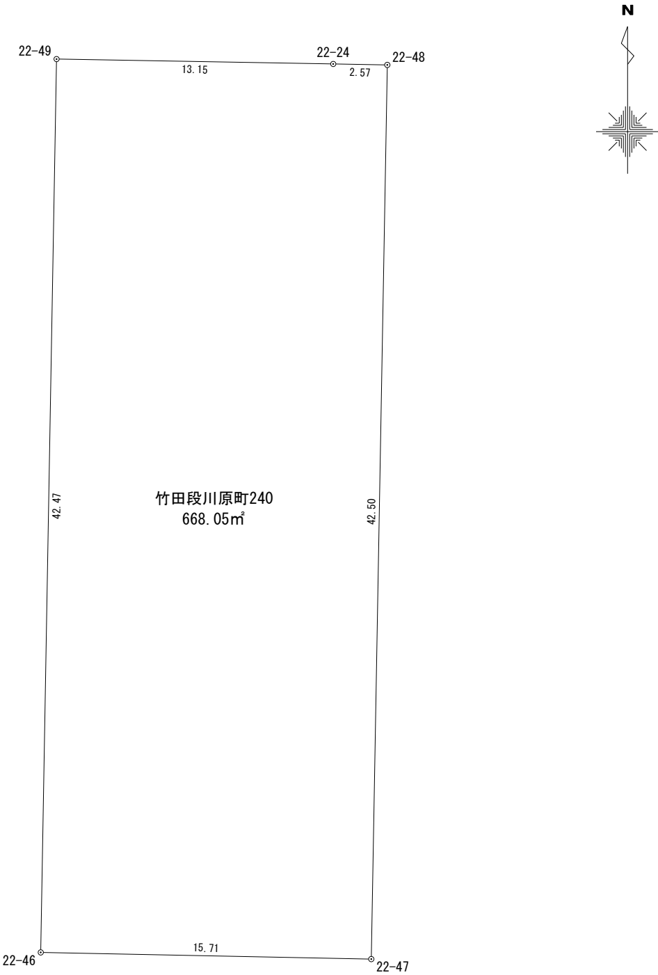
座 標 求 積 表
