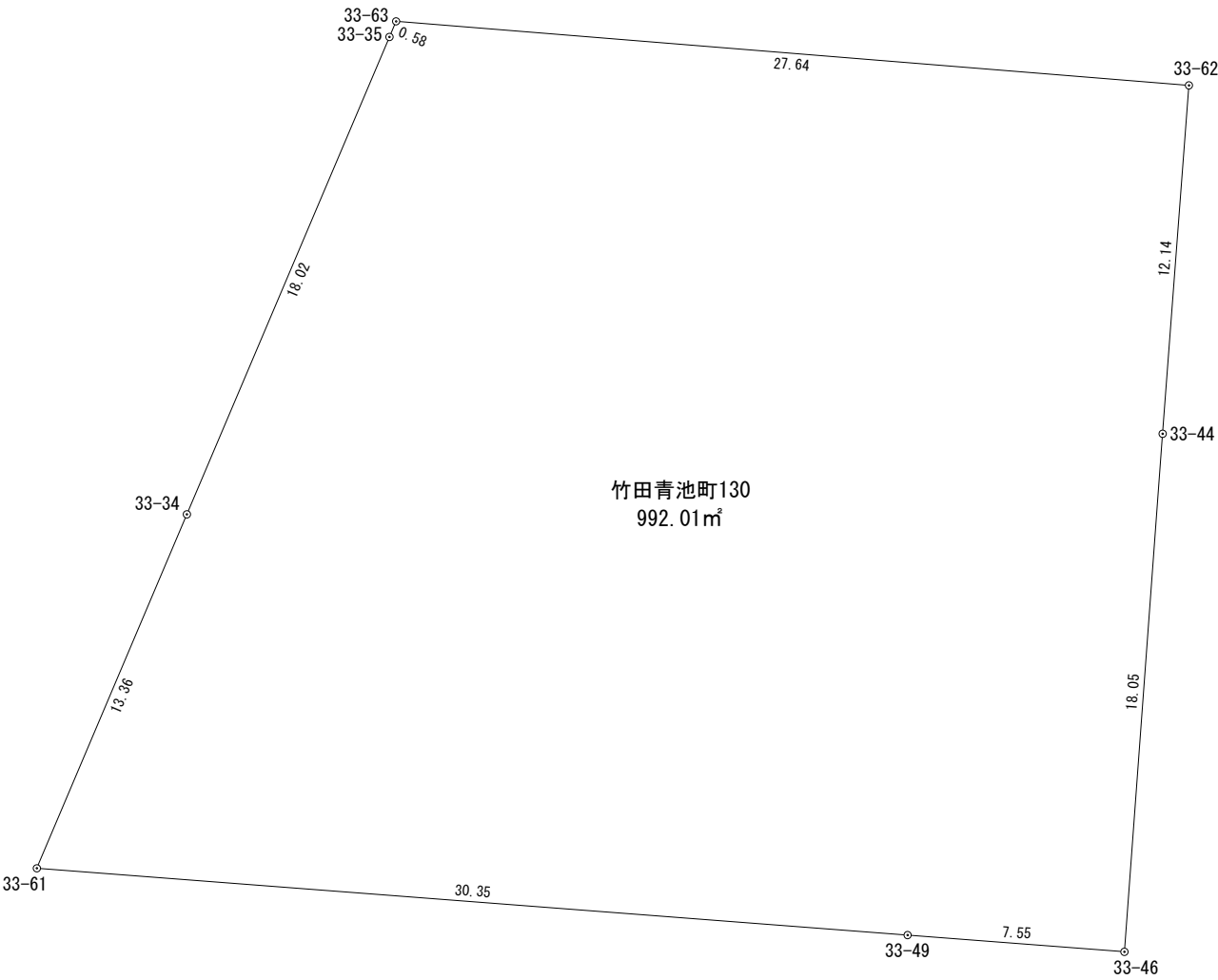
座 標 求 積 表
