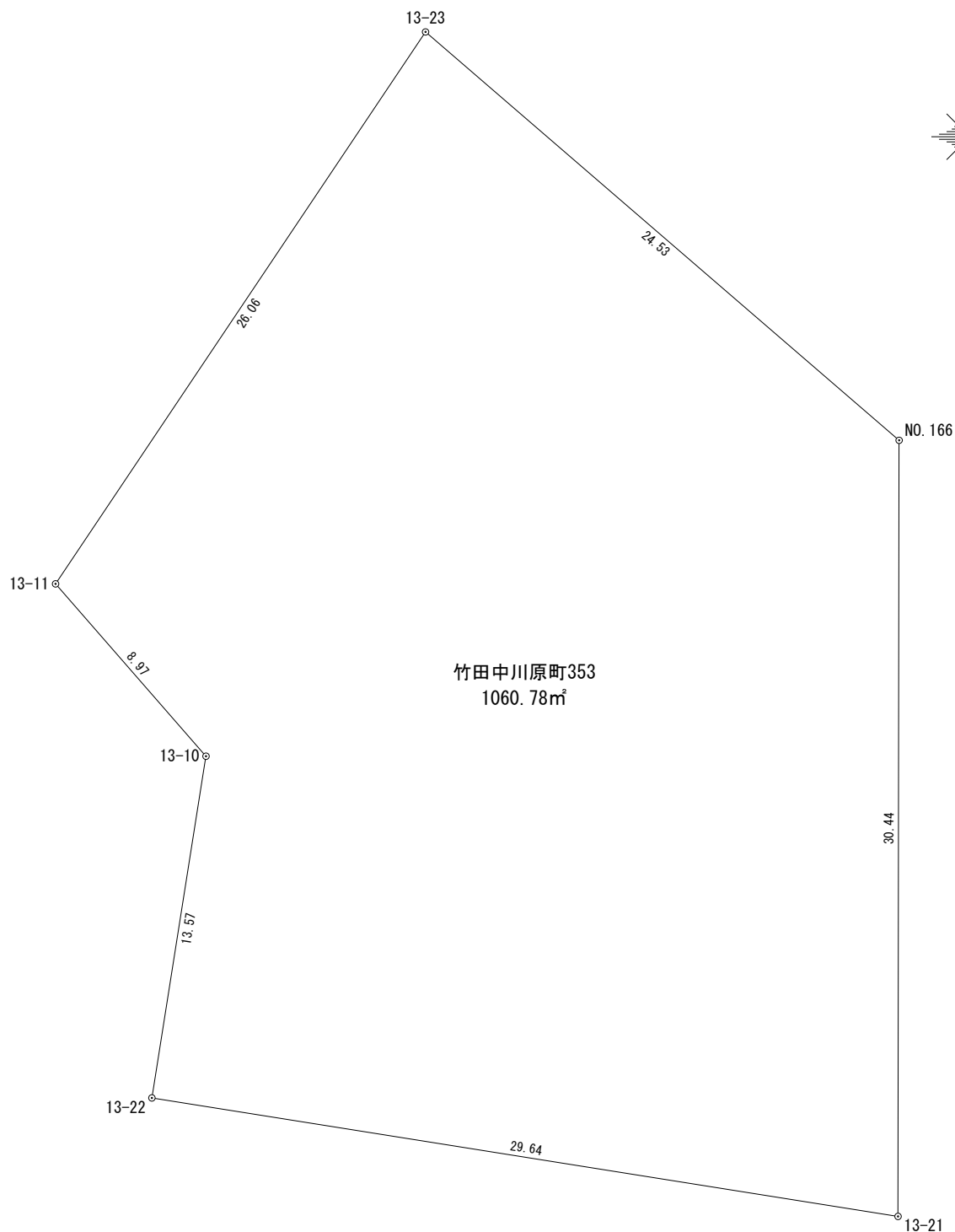
座 標 求 積 表
