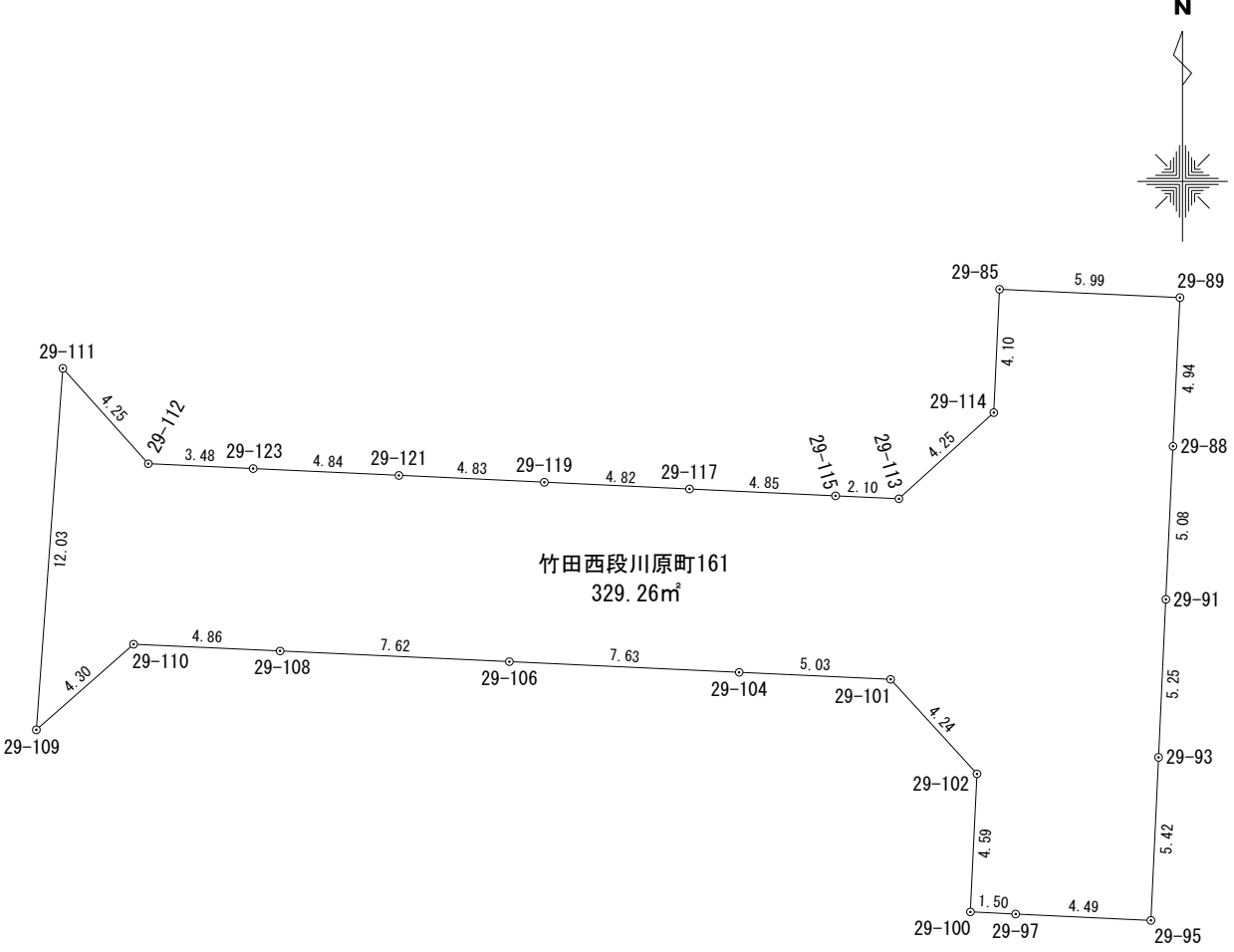
座 標 求 積 表
