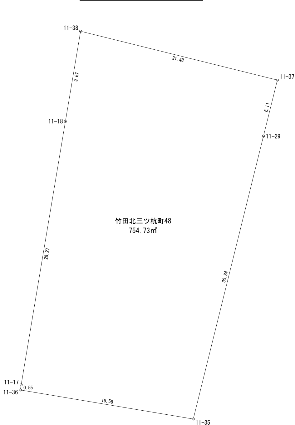
座 標 求 積 表
