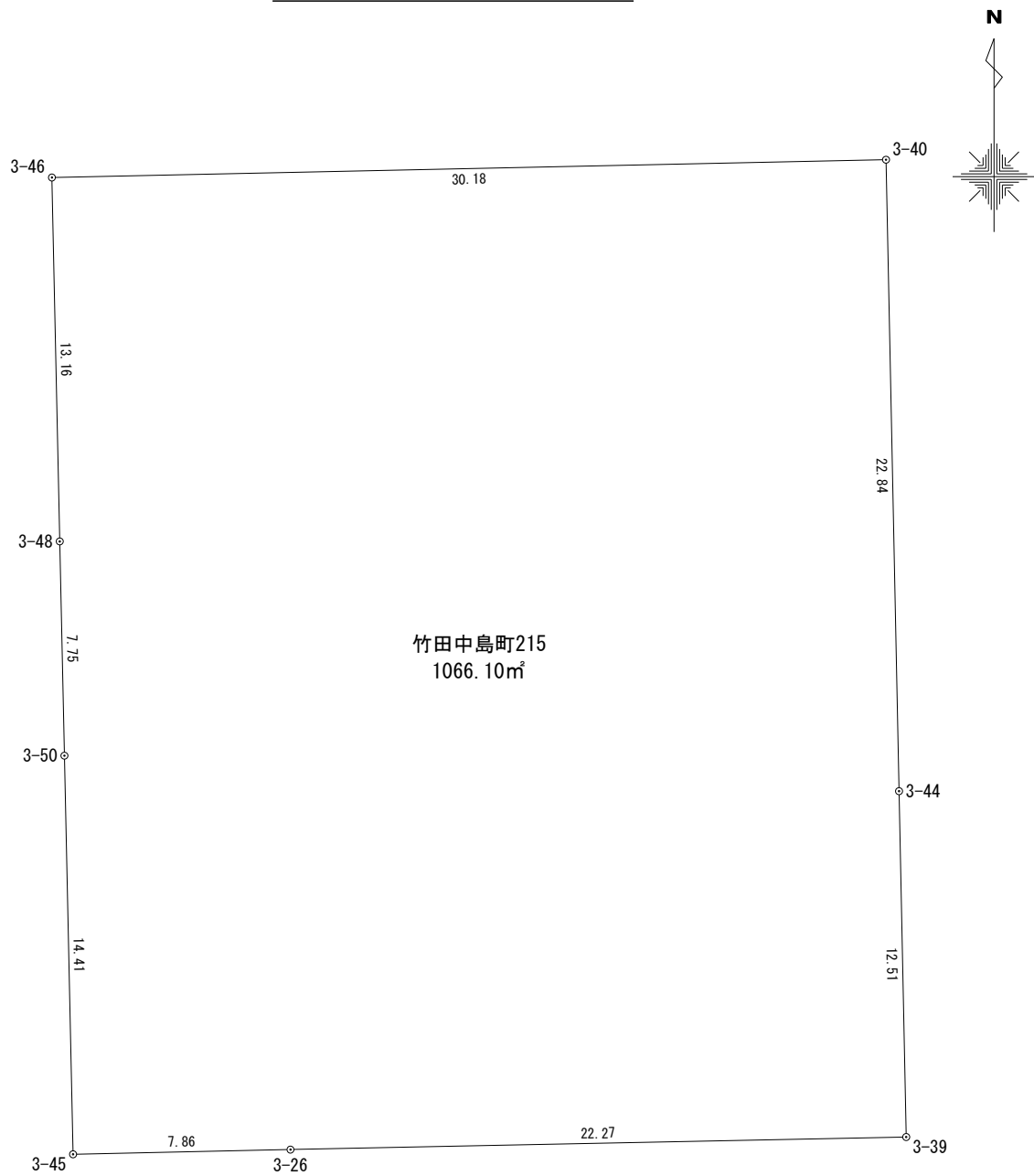
座 標 求 積 表
