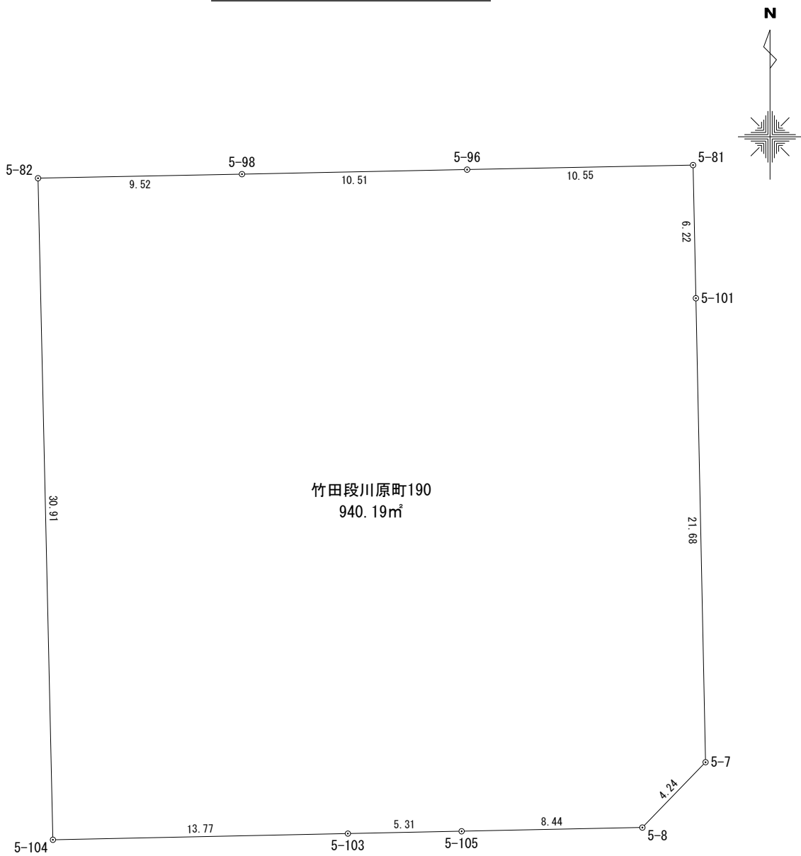
座 標 求 積 表
