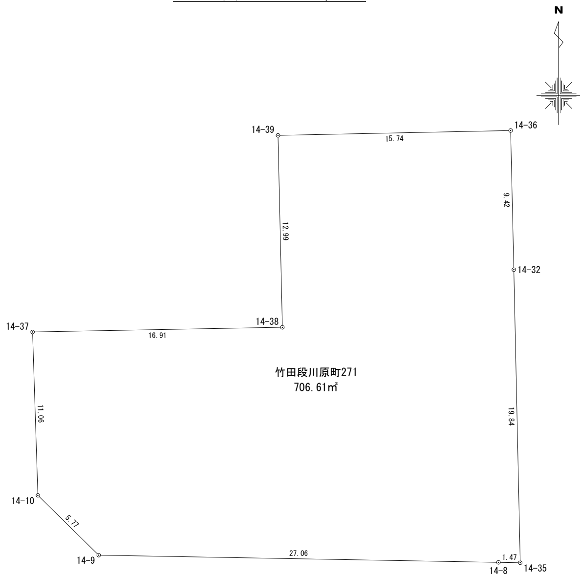
座 標 求 積 表
