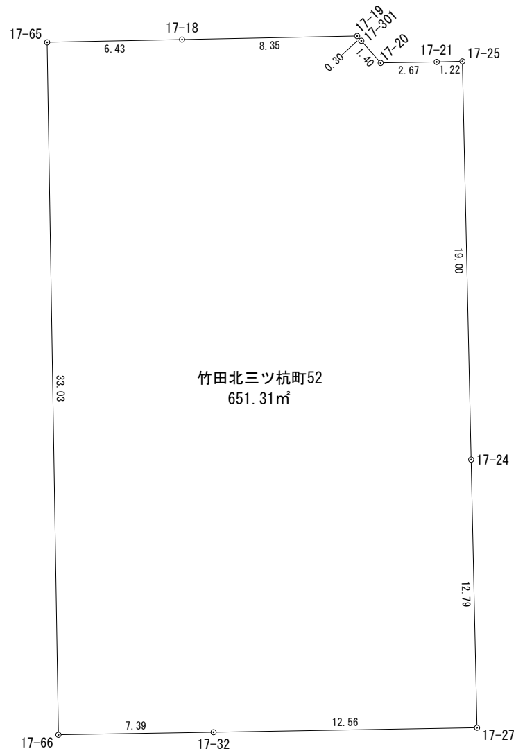
座 標 求 積 表
