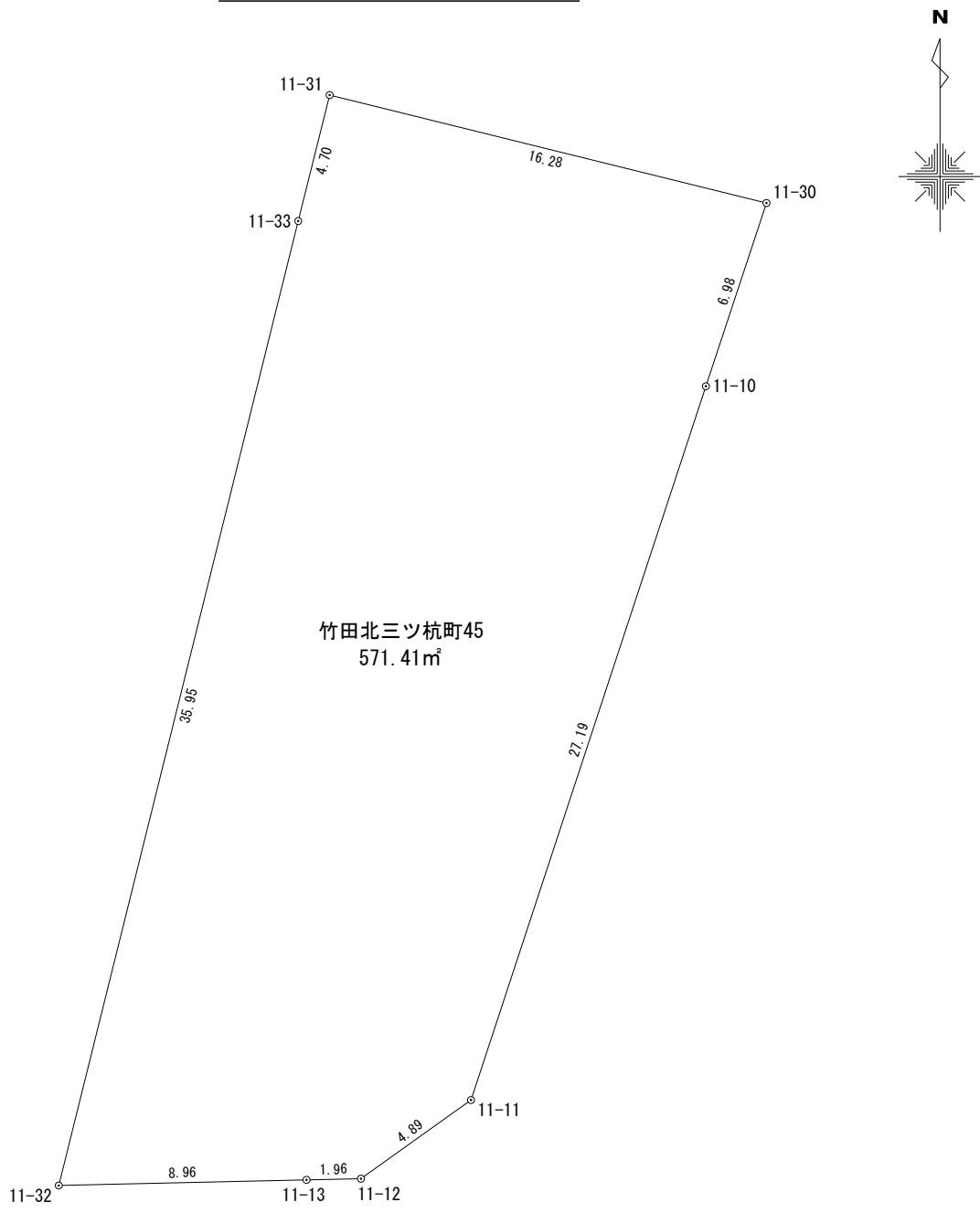
座 標 求 積 表
