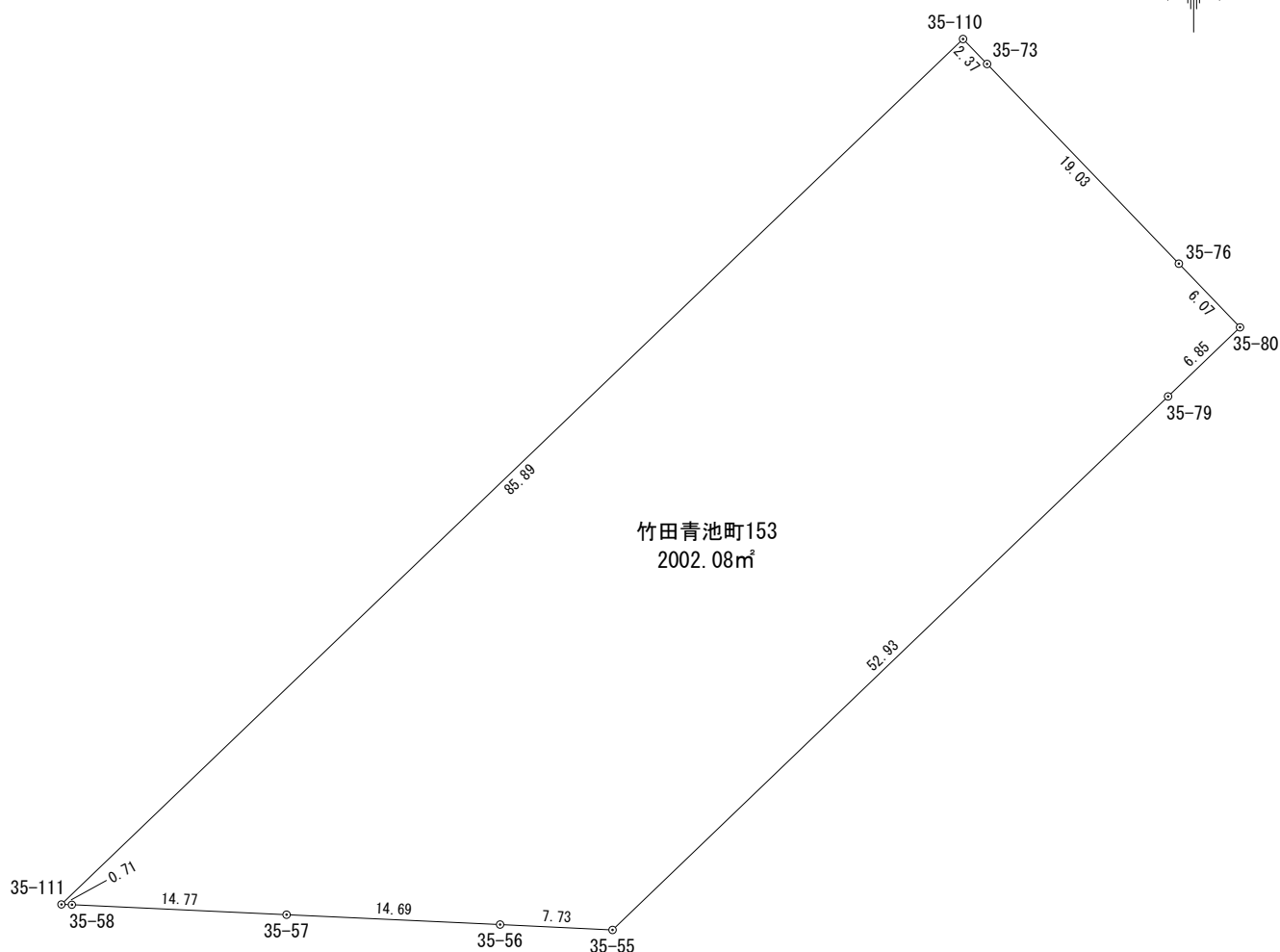
座 標 求 積 表
