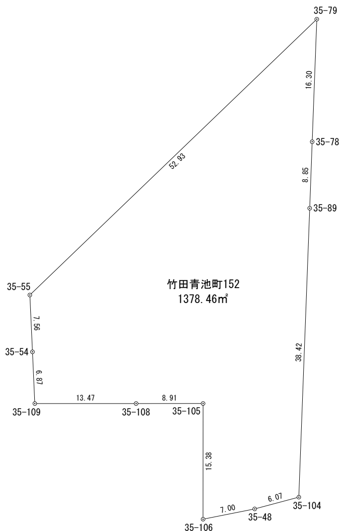
座 標 求 積 表
