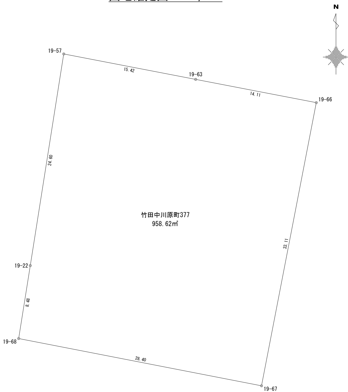
座 標 求 積 表
