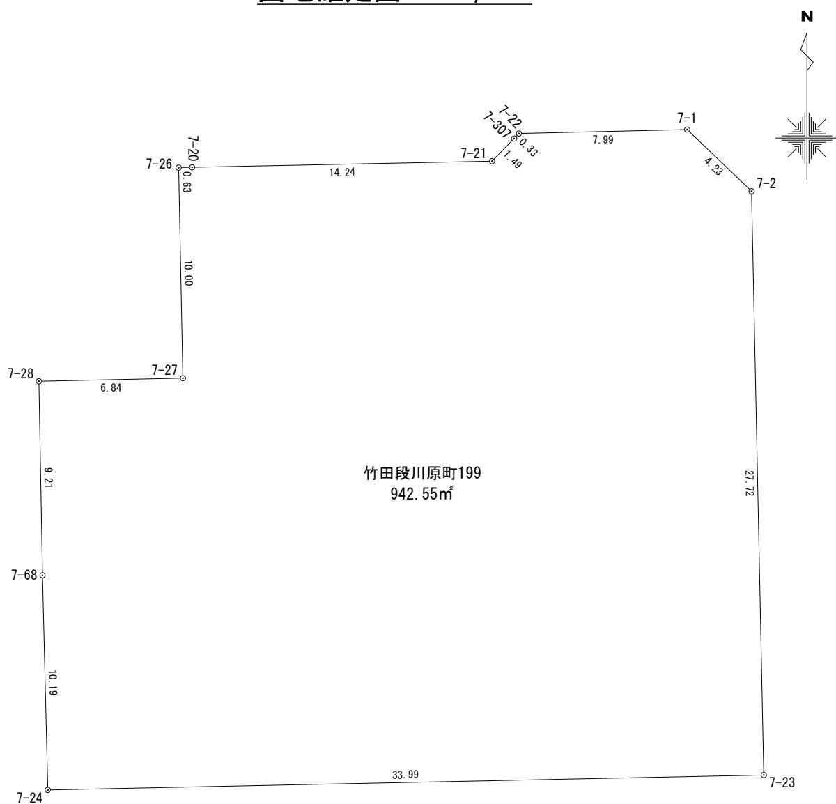
座 標 求 積 表
