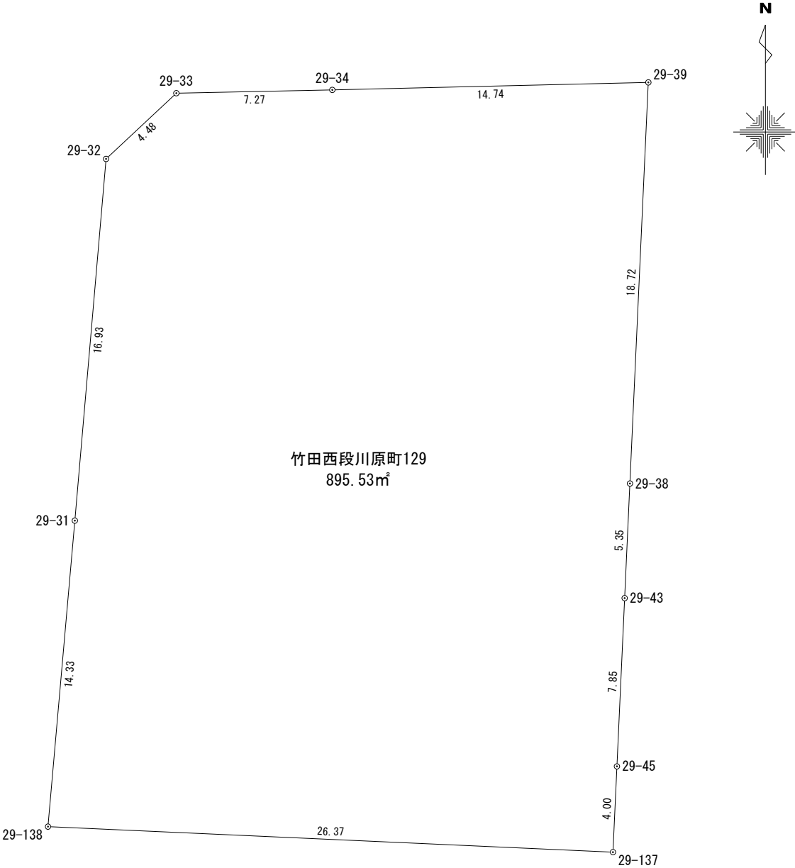
座 標 求 積 表
