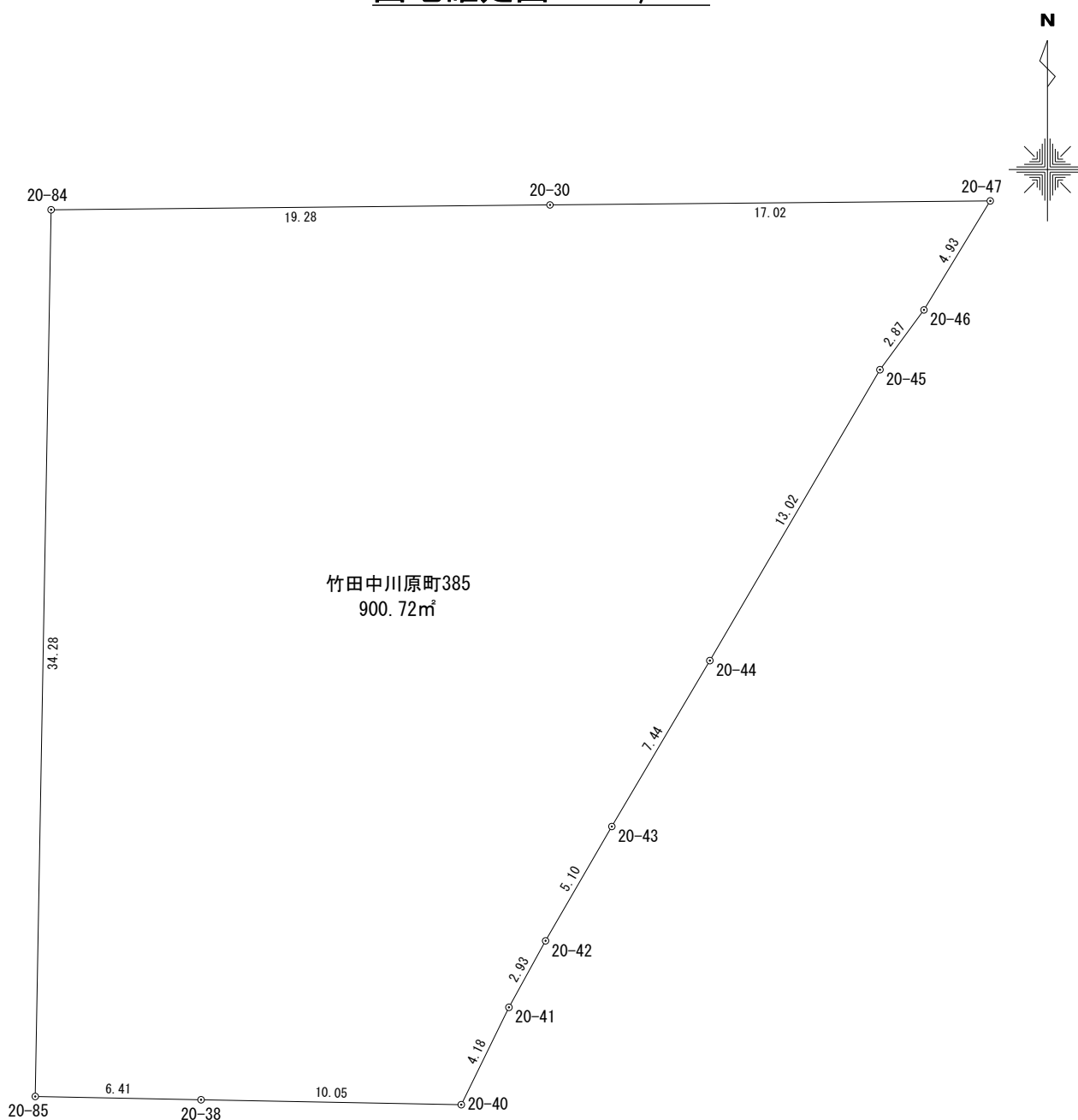
座 標 求 積 表
