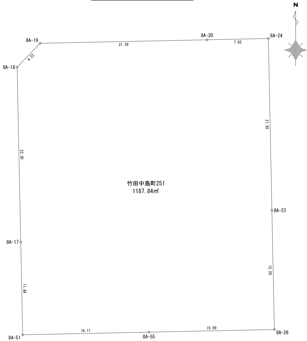
座 標 求 積 表
