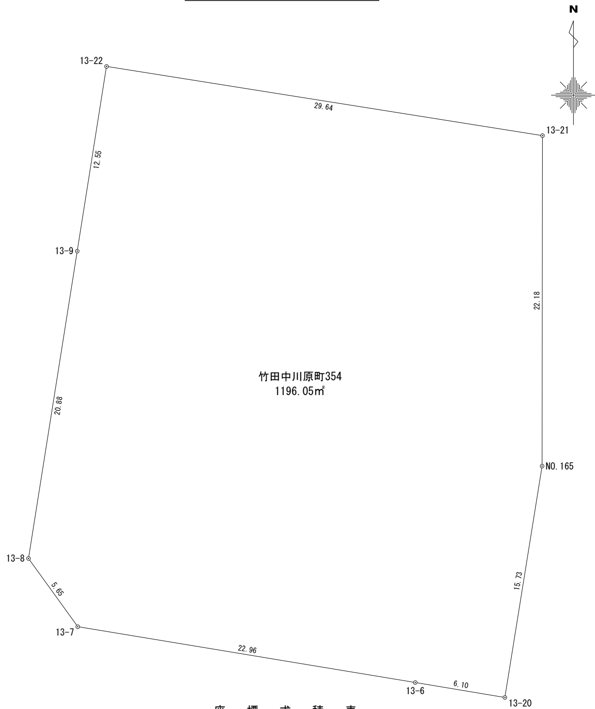
座 標 求 積 表
