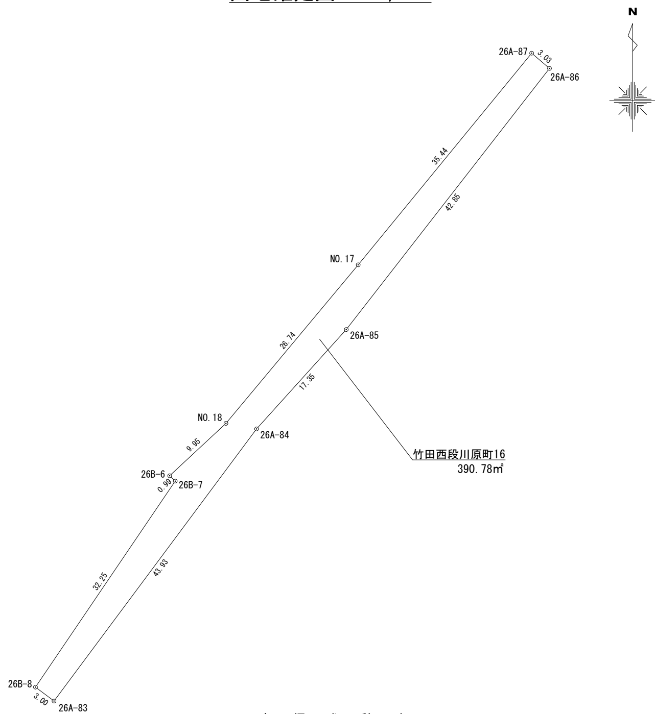
座 標 求 積 表
