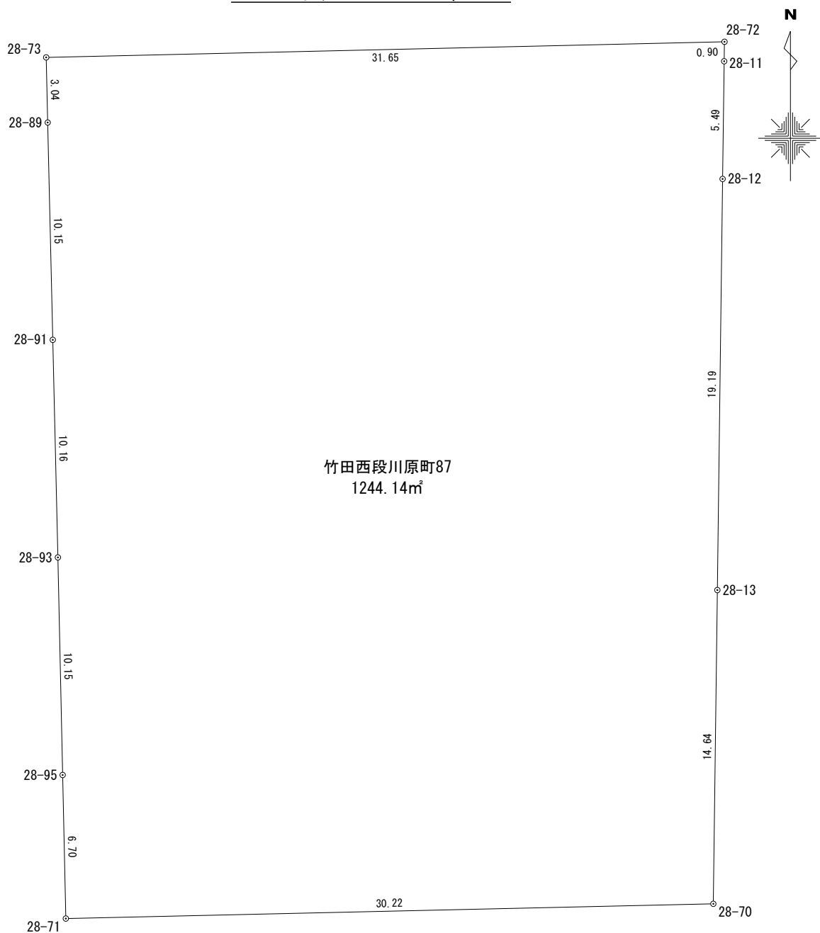
座 標 求 積 表
