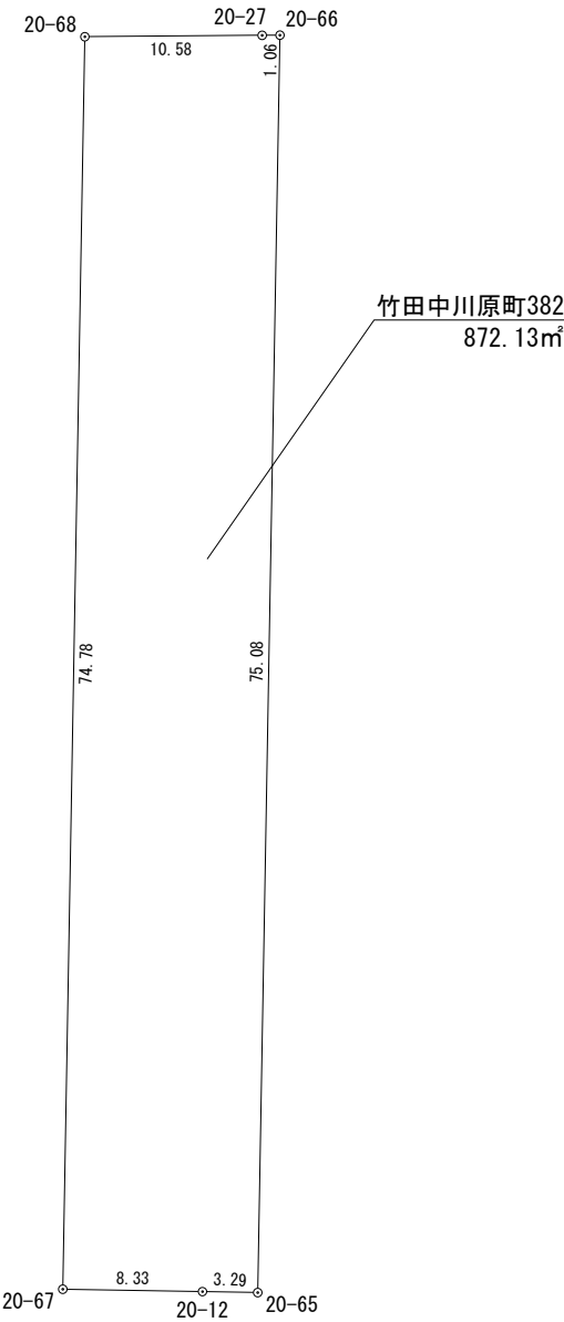
座 標 求 積 表
