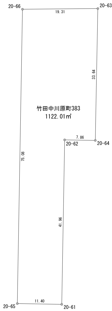
座 標 求 積 表
