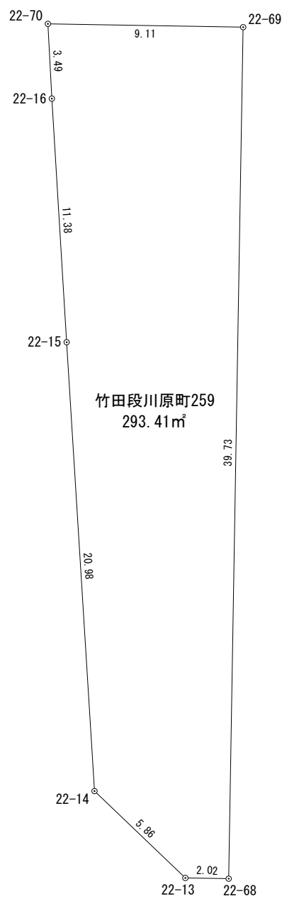
座 標 求 積 表
