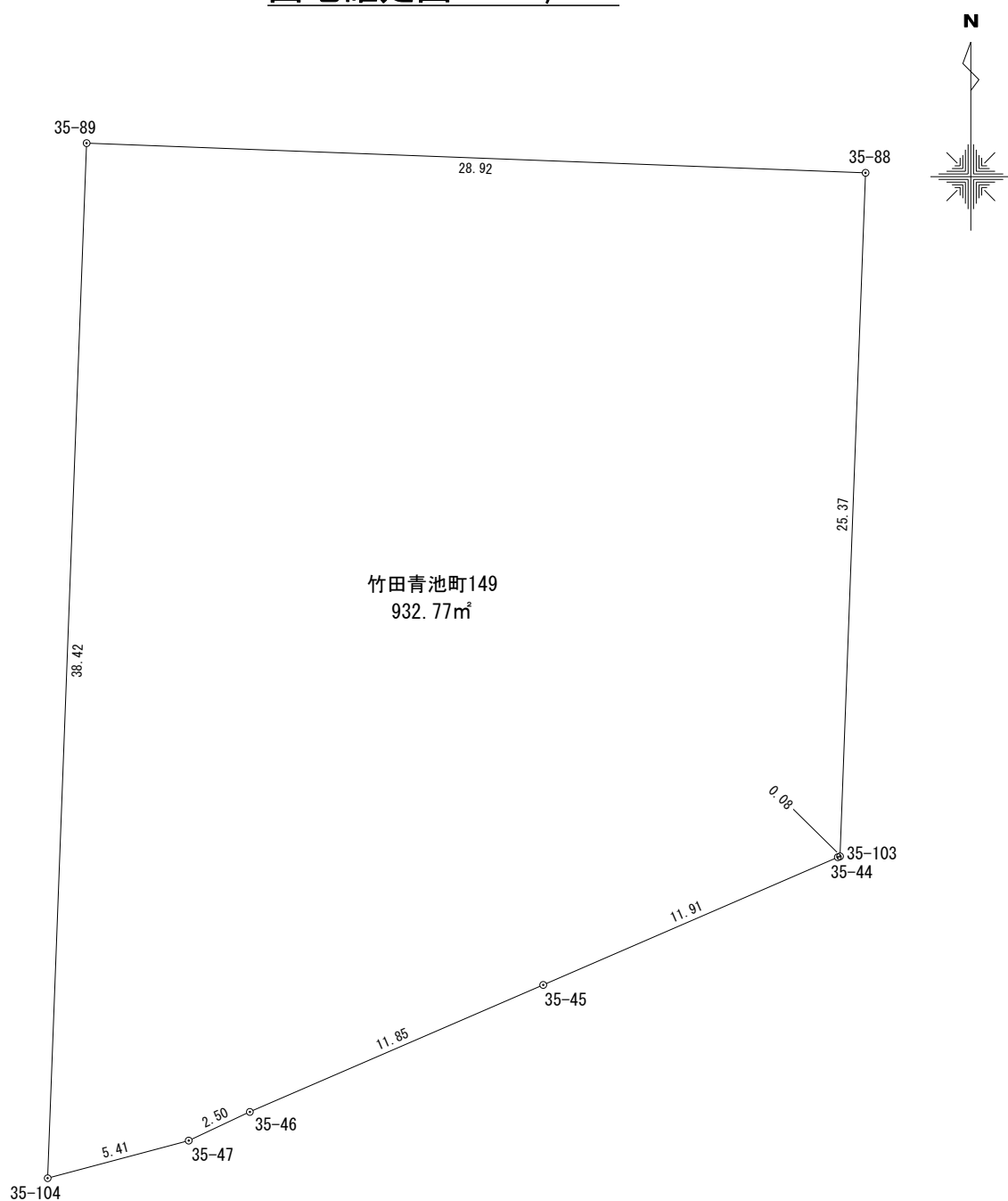
座 標 求 積 表
