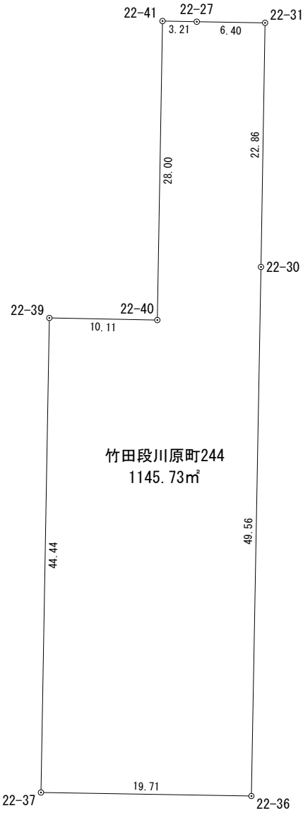
座 標 求 積 表
