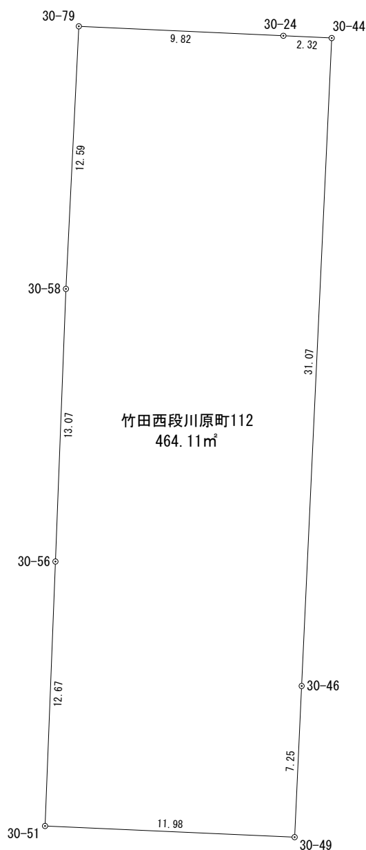
座 標 求 積 表
