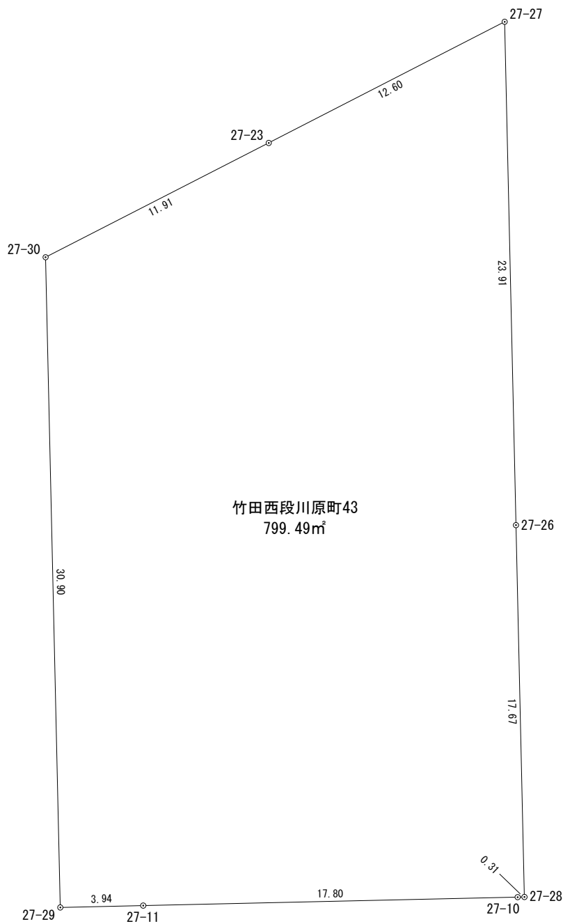
座 標 求 積 表
