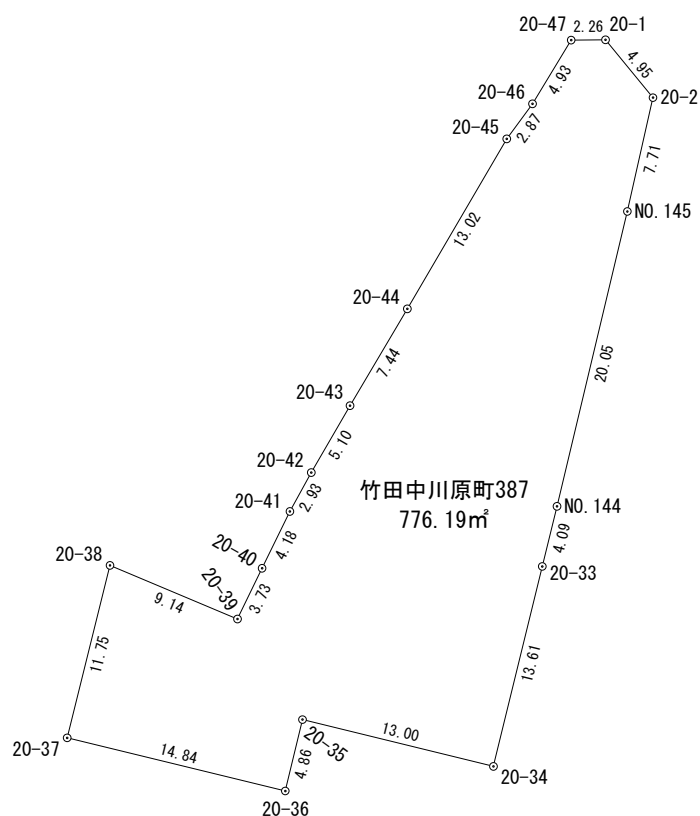
座 標 求 積 表
