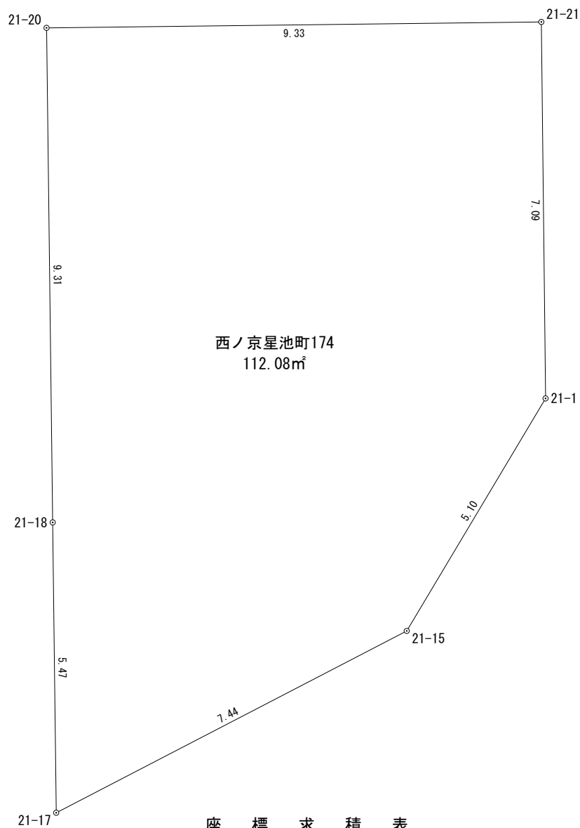
座 標 求 積 表
