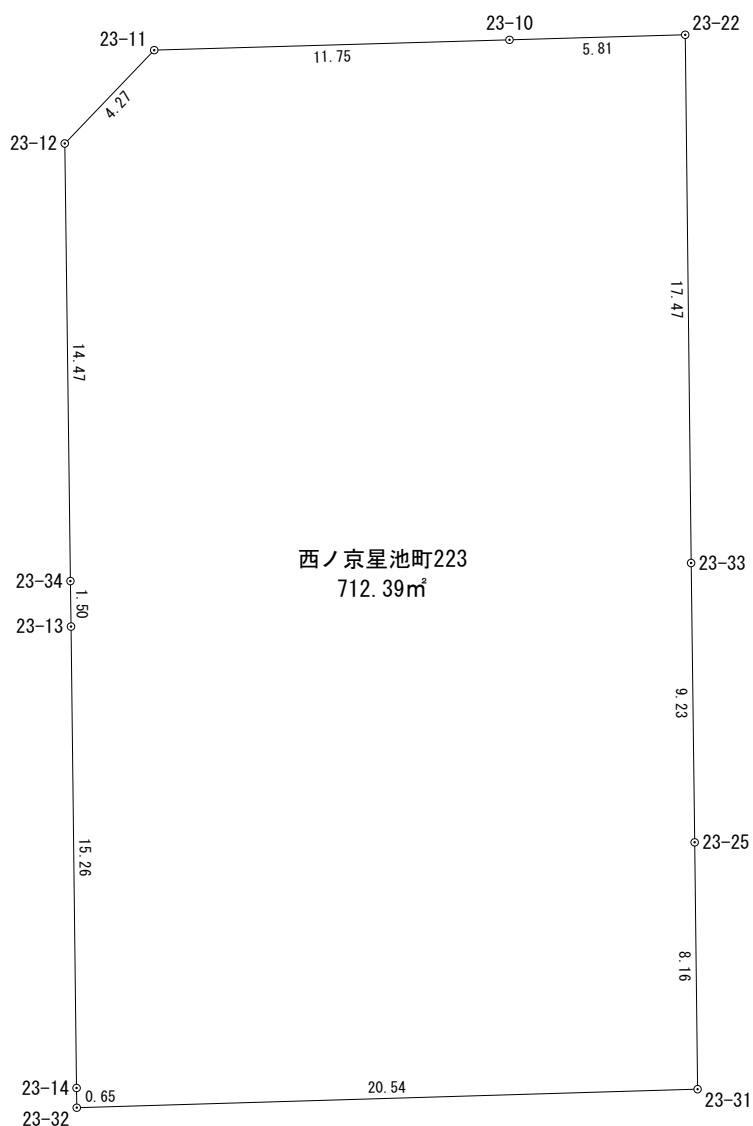
座 標 求 積 表
