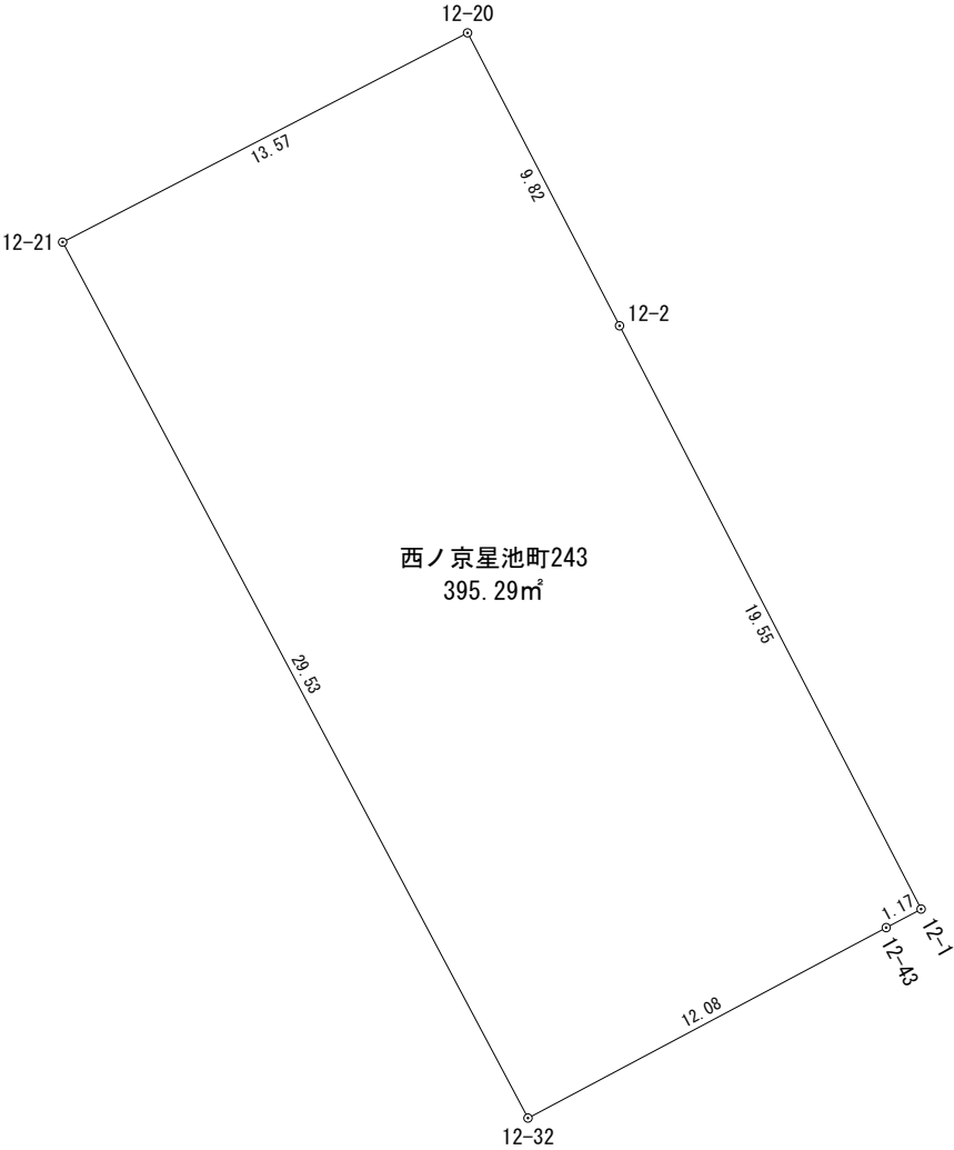
座 標 求 積 表
