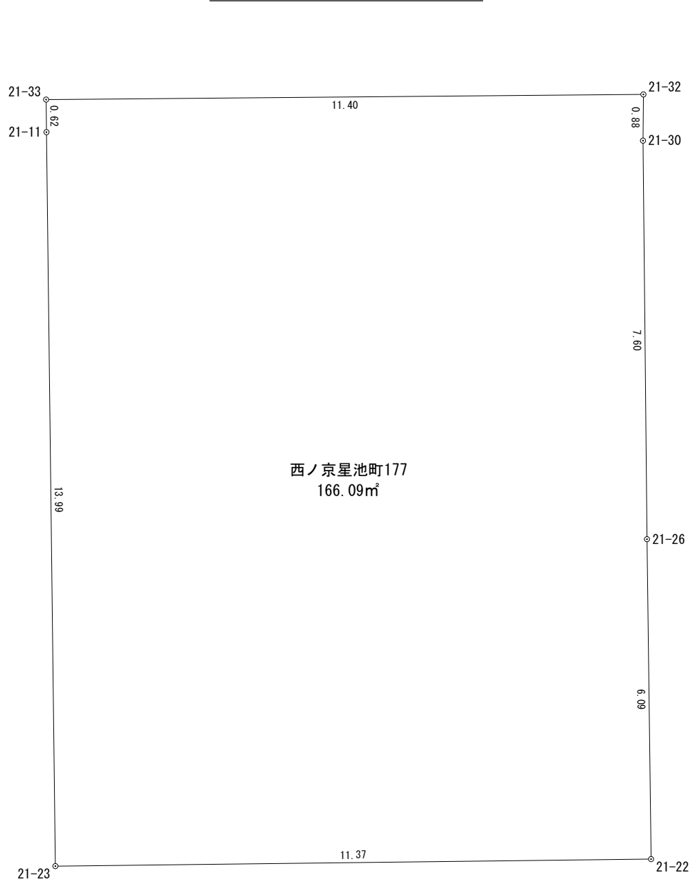
座 標 求 積 表
