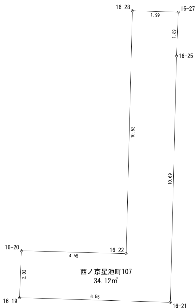
座 標 求 積 表
