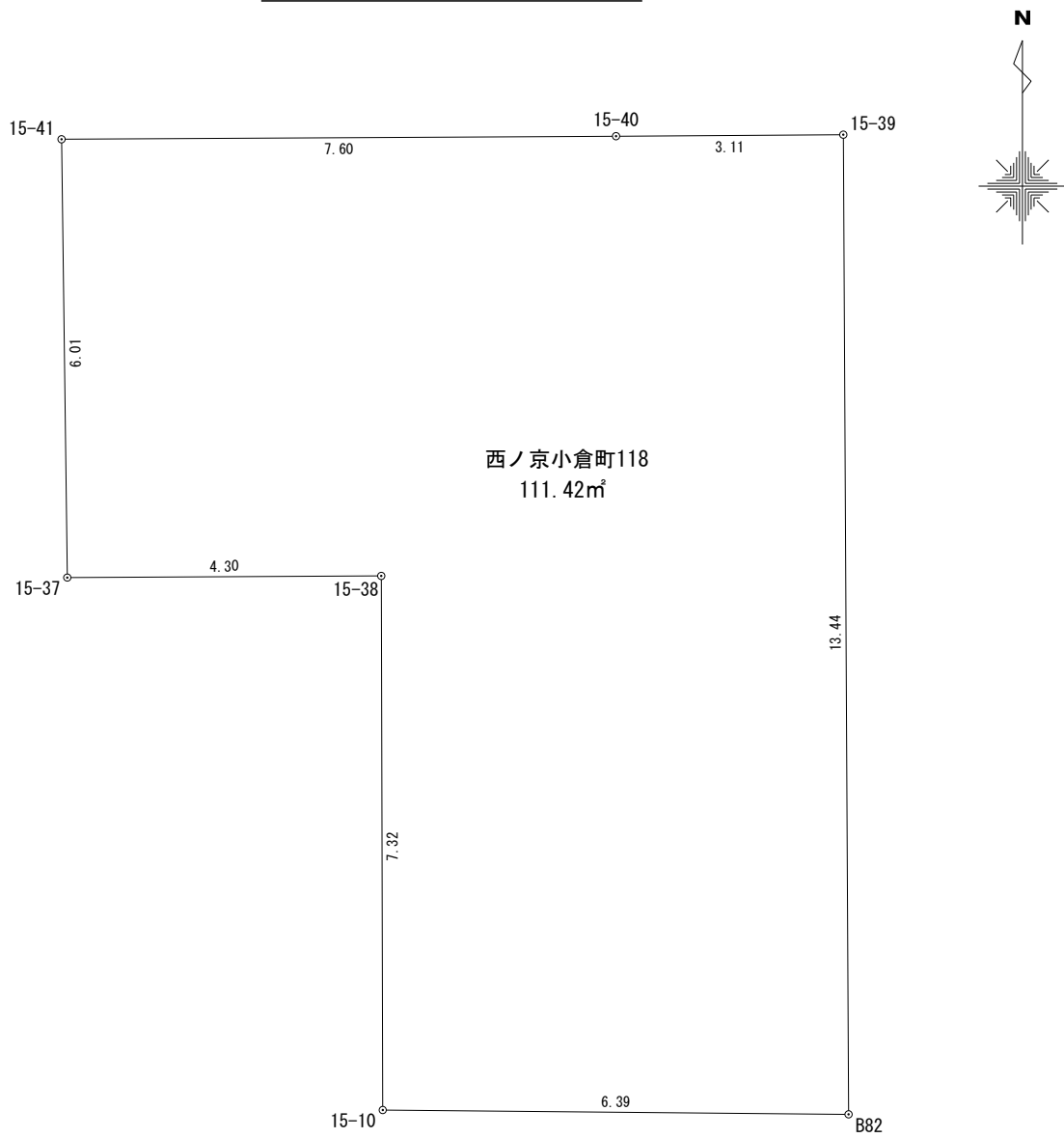
座 標 求 積 表
