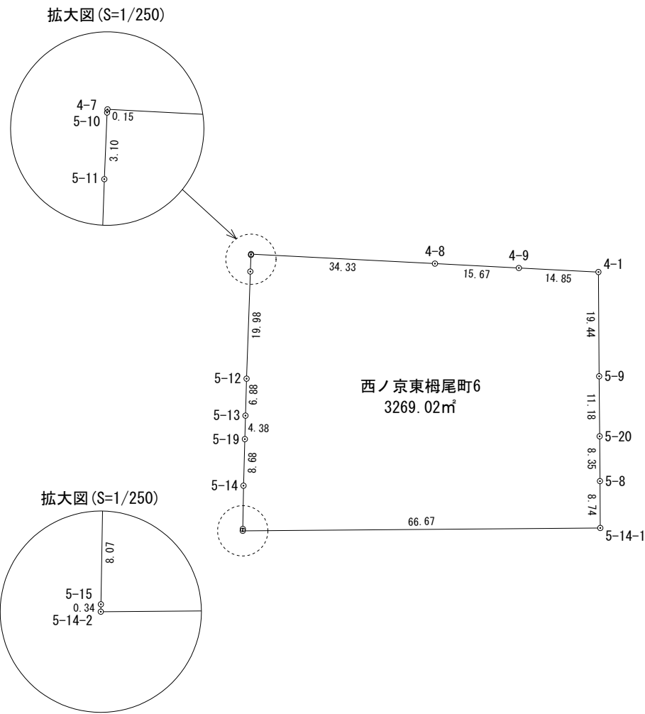
座 標 求 積 表
