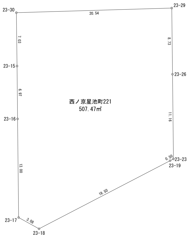
座 標 求 積 表
